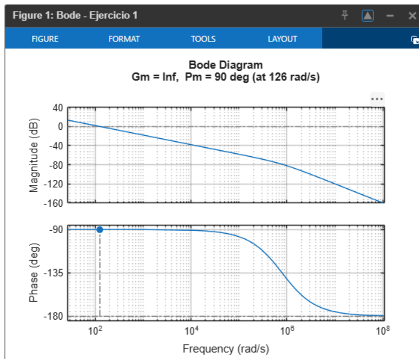
Figura 1. Diagrama de Bode del Ejercicio 1 (con márgenes). MATLAB: G_m = \text{Inf} , P_m = 90^\circ en 126 rad/s.
