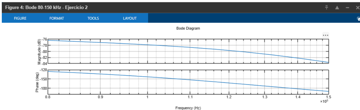
Figura 4. Diagrama de Bode del Ejercicio 2 en la banda de 80 kHz a 150 kHz.
