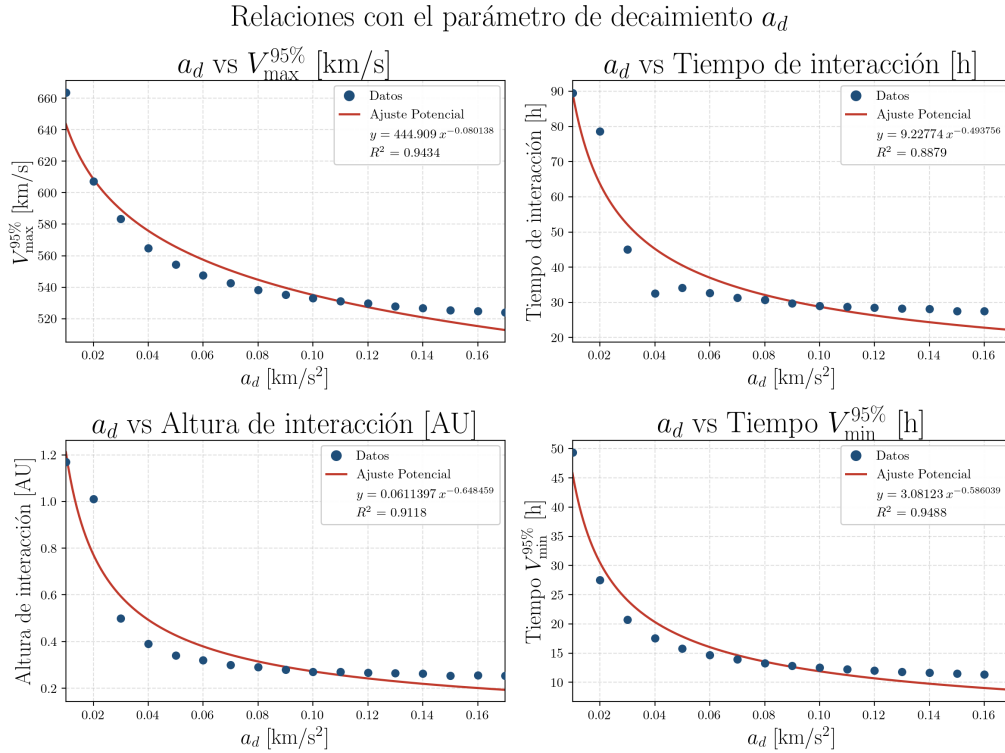
Figura 4.12: Gráficas de a_d vs parámetros de interacción, junto a las curvas de ajuste (línea roja) correspondientes y sus ecuaciones características. Los puntos en azul son los datos de la CME sucesora bajo los cuales ocurre la interacción. Además, se muestra su coeficiente de correlación.
