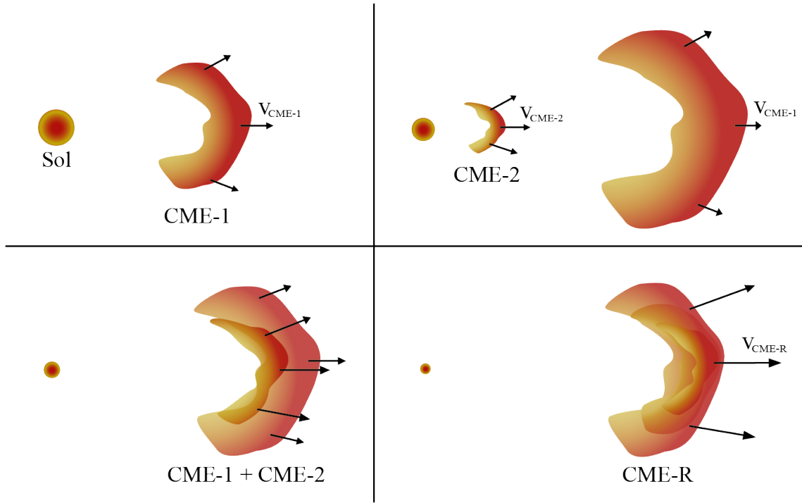
Figura 4.6: Bosquejo de interacción de CMEs con velocidades similares. La velocidad de la CME-1, v_{CME-1} es menor que la velocidad de la CME-2, v_{CME-2} , pero similar. Las densidades presentan una superposición, al igual que la velocidad, durante la interacción en el panel inferior derecho, produciendo una CME resultante con una velocidad y densidad mayores; tengase en cuenta el tamaño de los vectores velocidad y la opacidad en los colores de las CMEs.
