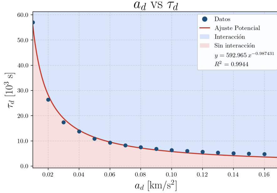
Figura 4.11: Gráfica de a_d vs \tau_d , junto a la curva de ajuste (línea roja) y su ecuación característica, la cual delimita una región de interacción (azul) de una región en donde no la hay (roja). Los puntos en azul son los datos de la CME sucesora bajo los cuales ocurre la interacción. Además, se muestra su coeficiente de correlación.
