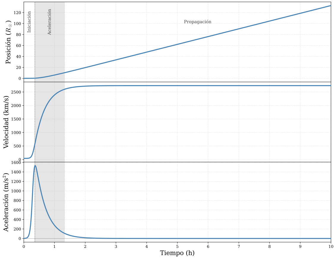
Figura 4.1: Perfiles de posición, velocidad y aceleración para la simulación de la CME inicial. Las diferentes etapas en la evolución de la CME se identifican con regiones delimitadas; la región de iniciación se indica en blanco hasta la línea discontinua, la etapa de aceleración se muestra en gris desde la línea discontinua hasta la punteada, la región de propagación en blanco va desde la línea punteada hasta el final de la gráfica. La línea discontinua indica el momento en el que la aceleración es máxima, mientras que la línea punteada señala el momento en el que la velocidad alcanza el 95 % de su velocidad máxima. Cabe señalar que el punto que se toma para determinar la cinemática de la CME es en su centro.
