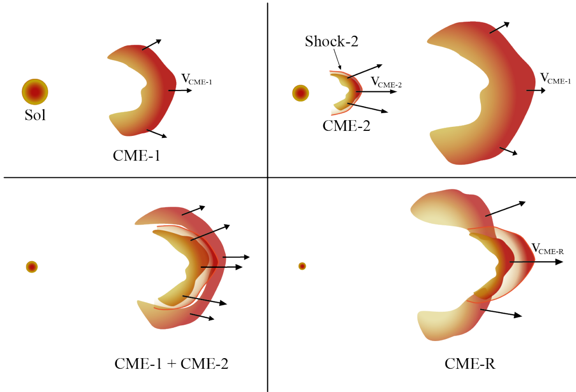
Figura 4.9: Bosquejo de interacción de CMEs con velocidades significativamente diferentes. La velocidad de la CME primaria, v_{CME-1} es mucho menor que la velocidad de la CME secundaria, v_{CME-2} . La CME-2 presenta un frente de onda de choque, puesto que su velocidad es super-Alfvénica, por lo que durante la interacción, en el panel inferior derecho, la CME-2 atraviesa abruptamente a la CME-1, debido a la diferencia entre sus velocidades. Tengase en cuenta el tamaño de los vectores velocidad y la opacidad en los colores de las CMEs.
