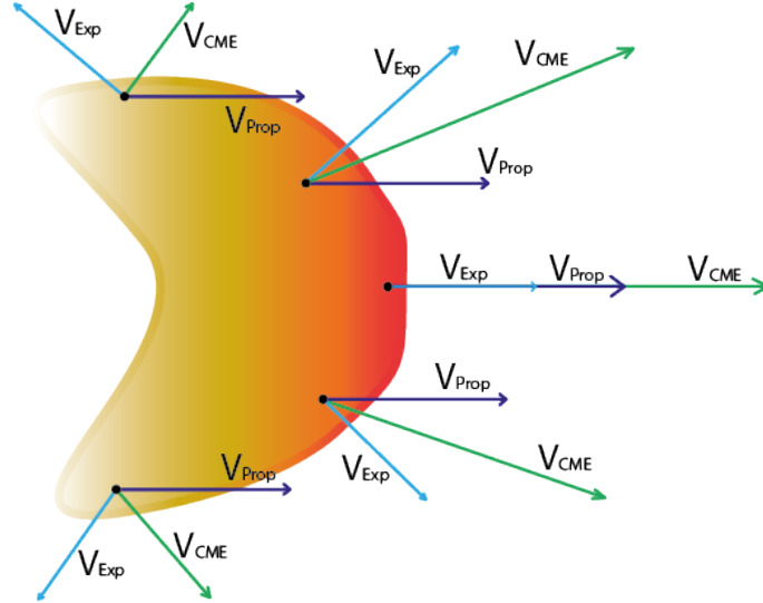
Figura 4.3: Representación del frente de una CME junto con los vectores de velocidad de propagación \vec{v}_{\text{Prop}} (azul oscuro) y de expansión \vec{v}_{\text{Exp}} (azul claro) en puntos cualquiera de la CME. El vector \vec{v}_{\text{Exp}} presenta direcciones hacia fuera de la CME en diferentes puntos, mientras que el vector \vec{v}_{\text{Prop}} tiene una dirección de propagación hacia la derecha en todo punto de la CME. Además, el vector resultante de la superposición del vector propagación y expansión, se muestra como \vec{v}_{\text{CME}} (verde) y cambia de dirección según el punto dentro de la CME.
