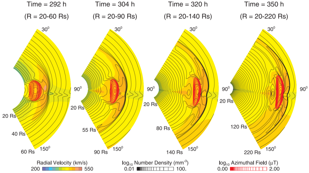
Figura 2.3: Propagación de una CME en la heliosfera, en donde la escala de colores muestra el mapa de velocidades, la densidad del plasma se muestra en relación a la densidad de líneas negras y el campo magnético en relación a la densidad de líneas rojas. Se muestra la evolución de la CME en 4 tiempos: 292, 304, 320 y 350 horas después de empezar a correr la simulación (Odstrcil et al., 2002)
