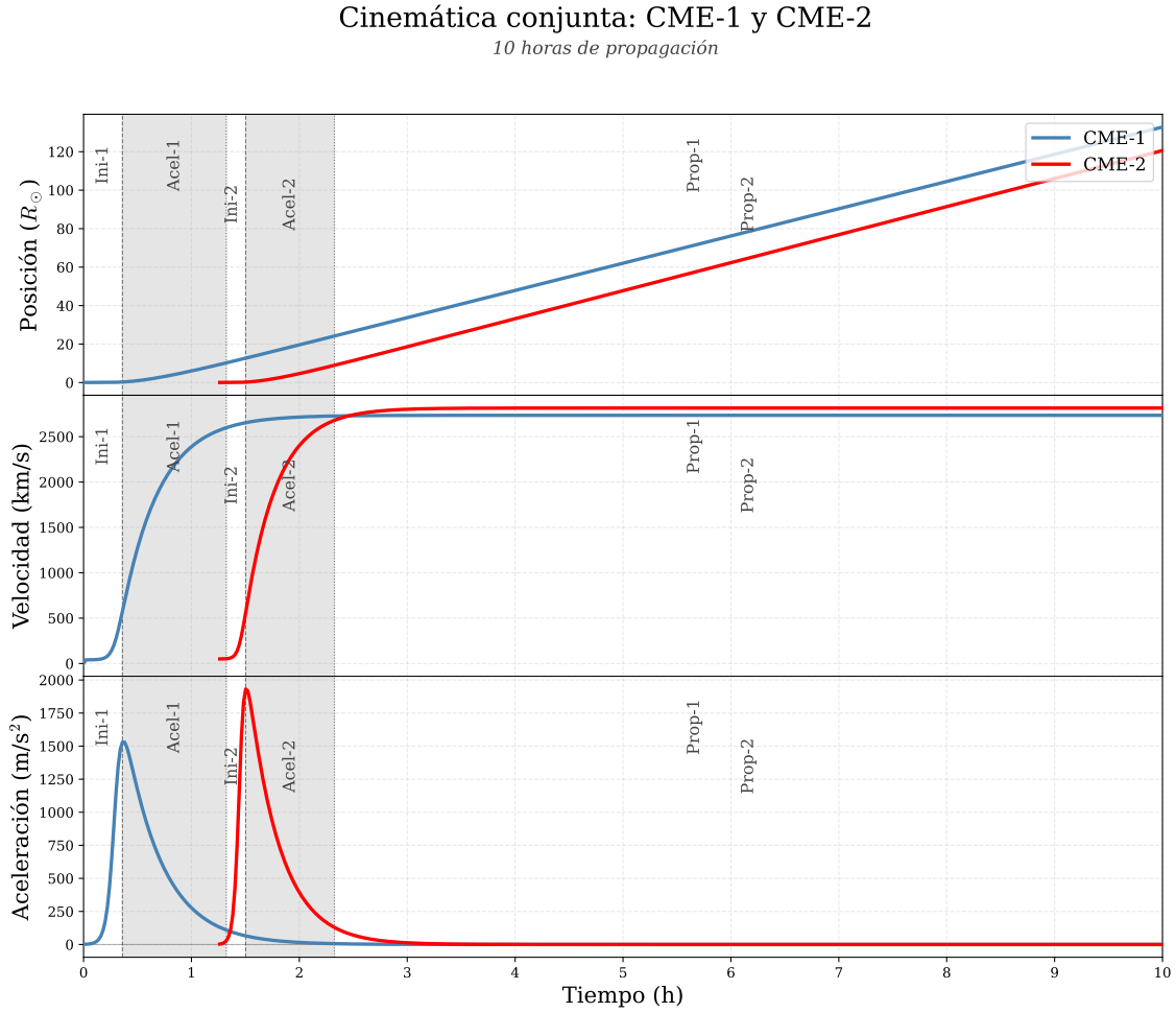
Figura 4.6: Perfiles cinemáticos de las dos CMEs sin considerar interacción. En azul se muestra la cinemática de la CME-1 y en rojo la de la CME-2, además se señalan las regiones de iniciación (blanco), aceleración (gris) y propagación (blanco) de las CMEs, etiquetadas con Ini, Acel y Prop. También, las etapas de iniciación y aceleración están separadas por una línea discontinua, mientras que las etapas de aceleración y propagación lo están con una línea punteada.
