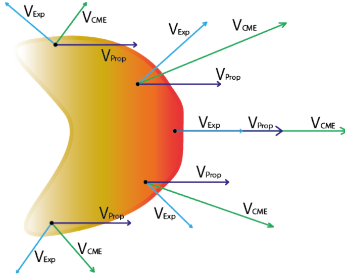
Figura 4.1: Representación del frente de una CME junto con los vectores de velocidad de propagación \vec{v}_{\text{Prop}} (azul oscuro) y de expansión \vec{v}_{\text{Exp}} (azul claro) en puntos cualquiera de la CME. El vector \vec{v}_{\text{Exp}} presenta direcciones hacia fuera de la CME en diferentes puntos, mientras que el vector \vec{v}_{\text{Prop}} tiene una dirección de propagación hacia la derecha en todo punto de la CME. Además, el vector resultante de la superposición del vector propagación y expansión, se muestra como \vec{v}_{\text{CME}} (verde) y cambia de dirección según el punto dentro de la CME.
