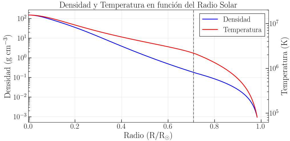
Figura 1.1: Distribución radial de densidad (azul) y temperatura (rojo) en el modelo solar estándar. La línea discontinua indica la ubicación de la tacoclina, en R = 0,71 R_{\odot} . Datos tomados de Software and Data for Solar Neutrino Research . Nota: Figura de elaboración propia.
