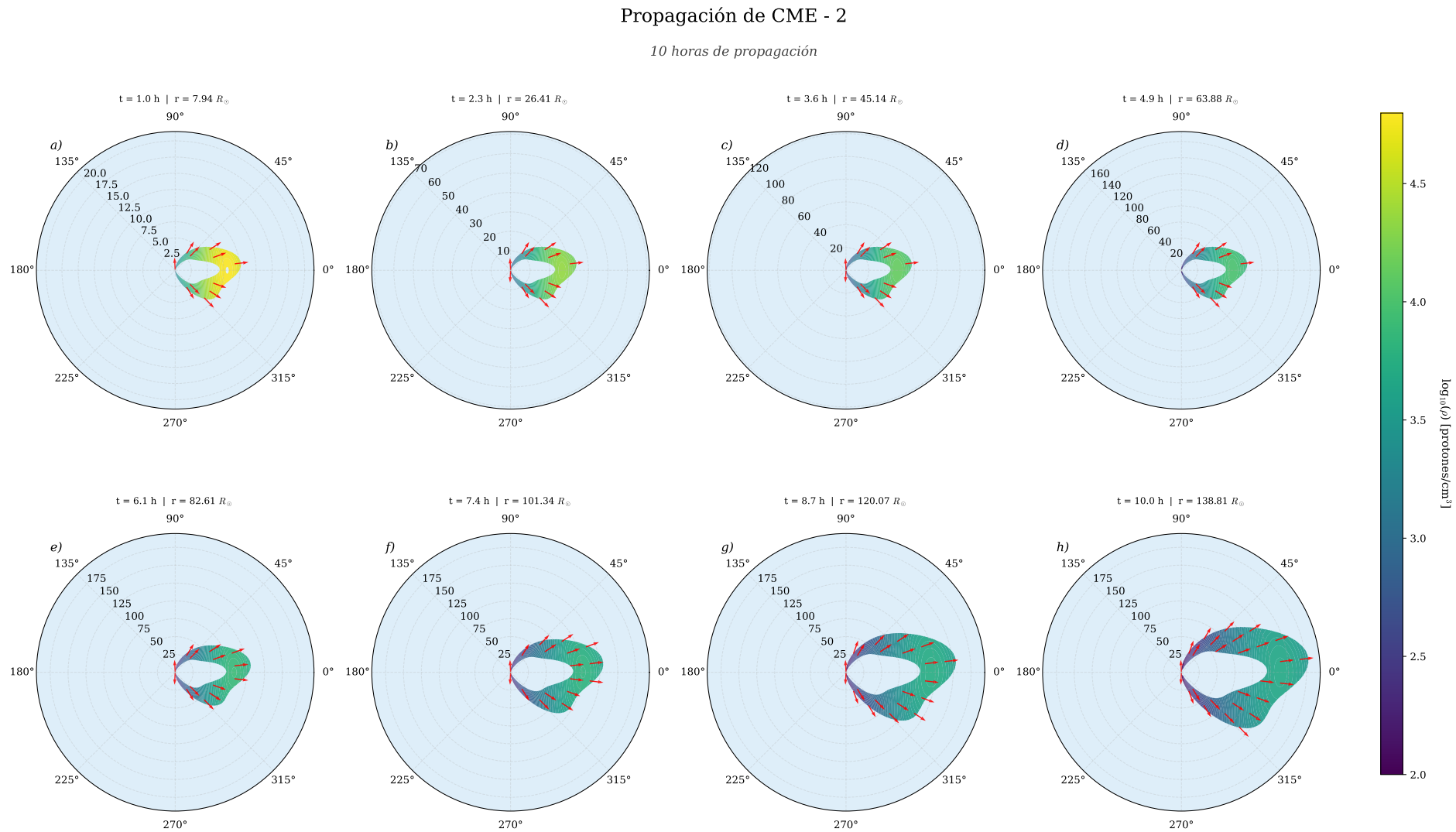
Figura 4.10: Evolución en 2D de la CME-2 durante 10 horas. La densidad se describe en escala de colores y la velocidad a través de un campo vectorial en rojo. En la parte superior de cada panel se indica el tiempo transcurrido y la posición del centro de la CME.
