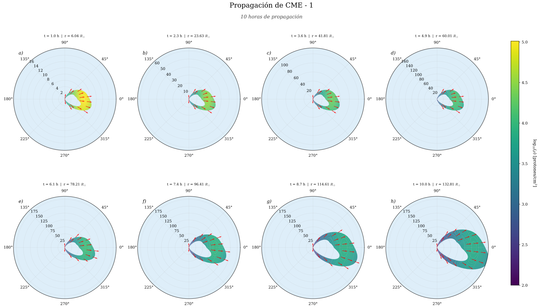
Figura 4.9: Evolución en 2D de la CME-1 durante 10 horas. La densidad se describe en escala de colores y la velocidad a través de un campo vectorial en rojo. En la parte superior de cada panel se indica el tiempo transcurrido y la posición del centro de la CME.
