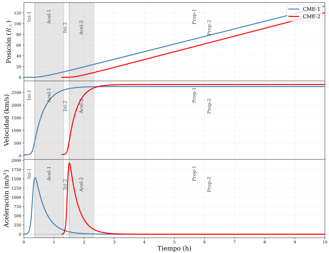
Figura 4.7: Perfiles cinemáticos de las dos CMEs sin considerar interacción. En azul se muestra la cinemática de la CME-1 y en rojo la de la CME-2, además se señalan las regiones de iniciación (blanco), aceleración (gris) y propagación (blanco) de las CMEs, etiquetadas con Ini, Acel y Prop. También, las etapas de iniciación y aceleración están separadas por una línea discontinua, mientras que las etapas de aceleración y propagación lo están con una línea punteada.
