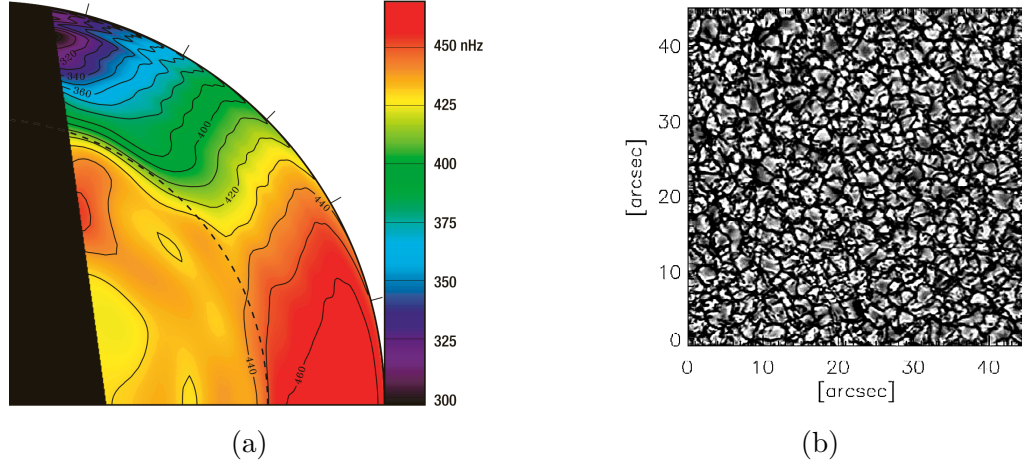
Figura 1.3: (a) Perfil de rotación interna solar obtenido con MDI/SOHO mediante inversión heliosísmica (método SOLA), en función de la profundidad radial y la latitud. El color indica la velocidad angular en nHz (rojo: rotación rápida; morado: rotación lenta), donde 1 nHz equivale a una rotación cada 36.5 días. Las líneas de contorno delimitan superficies de igual velocidad y la curva discontinua señala la tacoclina. Nota: Tomado de Schou et al. (1998) y Thompson et al. (2003). (b) Imagen obtenida con IMAx/Sunrise I (junio de 2009). Las estructuras brillantes y oscuras corresponden respectivamente a plasma ascendente y descendente de la granulación solar. FOV: \sim 35 \times 35 Mm; resolución espacial: \sim 100 km \text{píxel}^{-1} . Nota: Tomado de Solanki et al. (2010).
