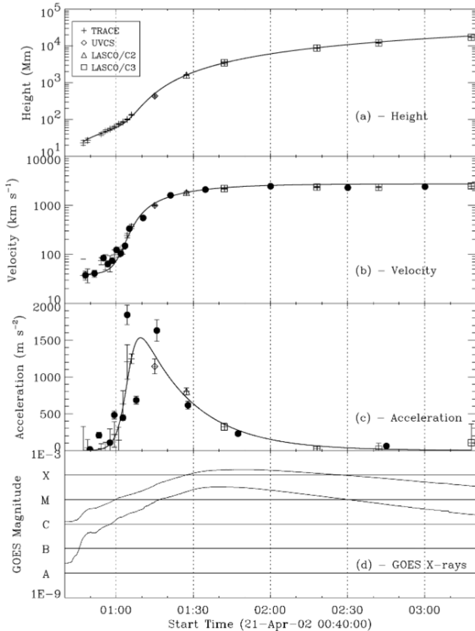
Figura 2.6: Perfil de altura, velocidad y aceleración de la CME del 21 de abril de 2002 a las 00:43 UT, en función del tiempo. Así mismo, el flujo de rayos X debido a su Flare asociada, en función del tiempo. Los círculos rellenos son valores derivados de la gráfica de altura vs tiempo, los demás símbolos señalan las observaciones del
