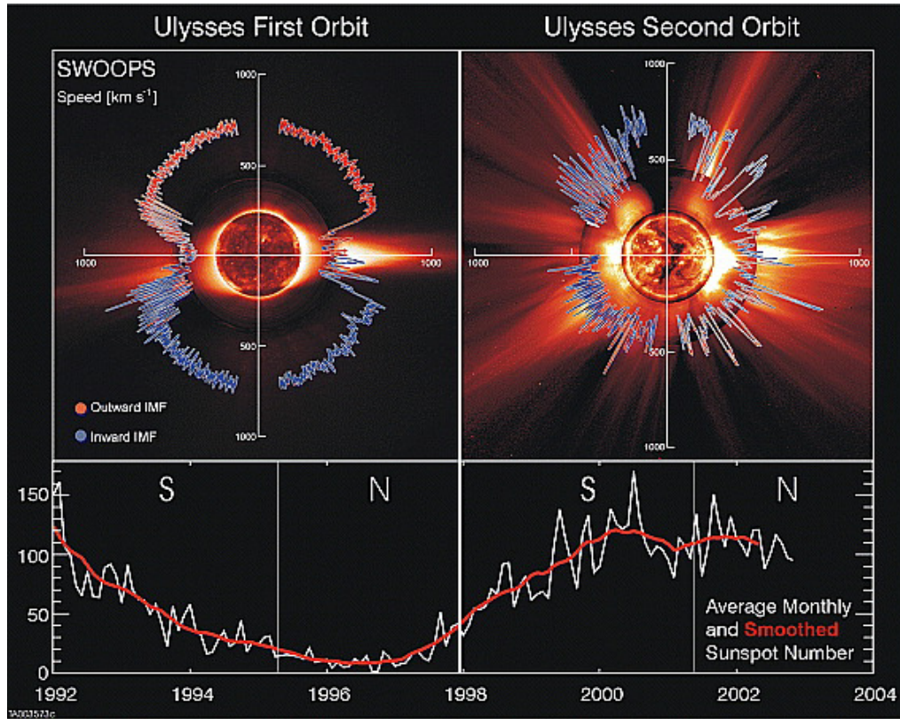
Figura 1.8: Gráficos polares de la velocidad del viento solar en función de la latitud para las dos primeras órbitas de Ulysses. Paneles superiores: Velocidad del viento solar medida por el instrumento SWOOPS , codificada por color según la polaridad del IMF , en rojo se indica un IMF hacia afuera (positivo) y en azul un IMF hacia adentro (negativo). Ambas se representan sobre imágenes solares compuestas características del mínimo solar (17/08/1996) y el máximo solar (07/12/2000). Paneles inferiores: Latitud heliográfica de Ulysses durante su órbita única de alta inclinación alrededor del Sol. El número de manchas (panel inferior) muestra que la primera órbita se produjo durante el mínimo del ciclo solar, mientras que la segunda abarcó el máximo solar. Tomado de McComas et al. (2003)
