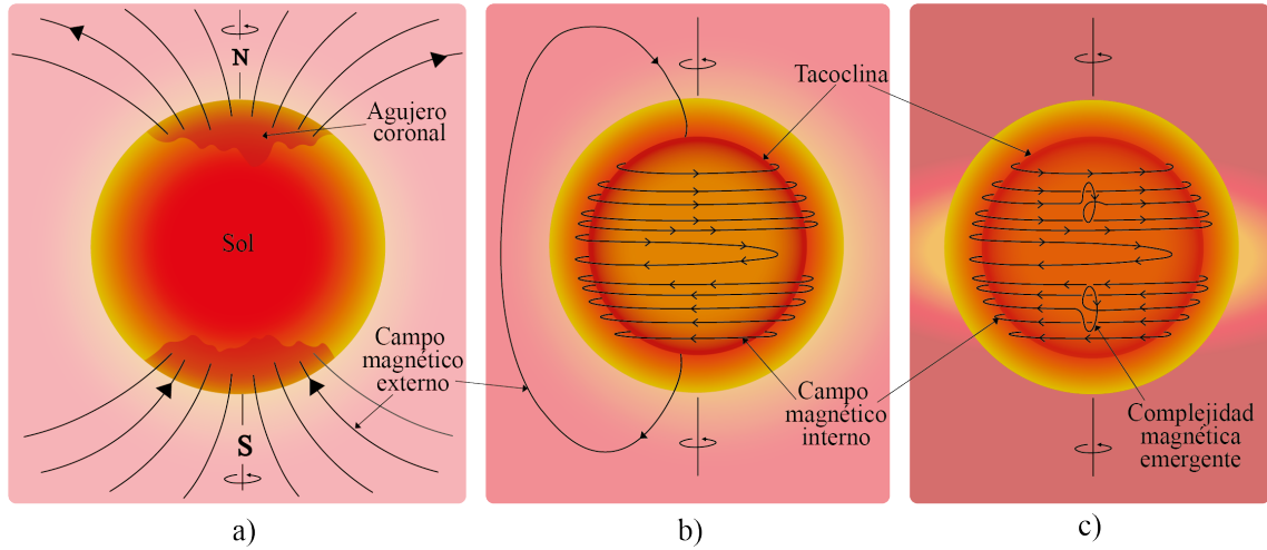
Figura 1.4: Comportamiento poloidal y toroidal del campo magnético del Sol. El panel a) muestra campos poloidales, un polo norte y un polo sur con líneas de campo magnético abiertas; el b) muestra su conversión interna en campos toroidales mediante el efecto \Omega , produciendo líneas de campo que envuelven el eje de rotación y sobre la tacoclina. El panel c) muestra el campo magnético emergente en forma de bucles a través de la superficie, regenerando el campo poloidal mediante el efecto \alpha .
