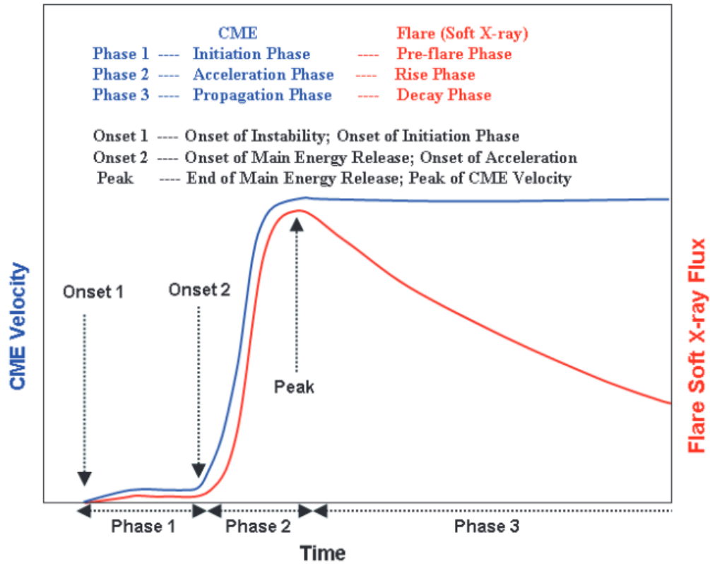
Figura 2.5: Perfil de aceleración de una CME y de su Flare asociada, mostrados como sus velocidades en función del tiempo. Se muestran las tres fases de la dinámica de la CME y de la Flare (e.g., Zhang & Dere, 2006).
