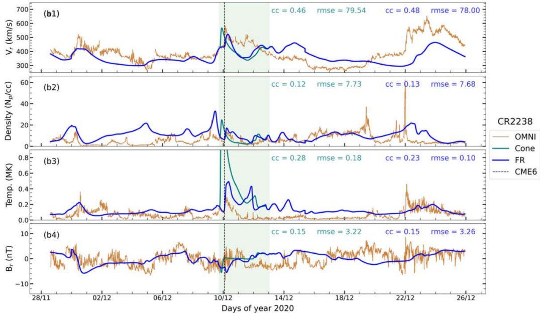
Figura 2.8: Gráficas de velocidad radial ( V_R ), densidad, temperatura y campo magnético radial ( B_r ), tomados de OMNI (línea naranja) y de las simulaciones: Cono elíptico (línea verde) y Cuerda de flujo (línea azul). También, la línea punteada indica la llegada de la CME, que en el paper llaman CME6. (Mayank et al., 2023)
