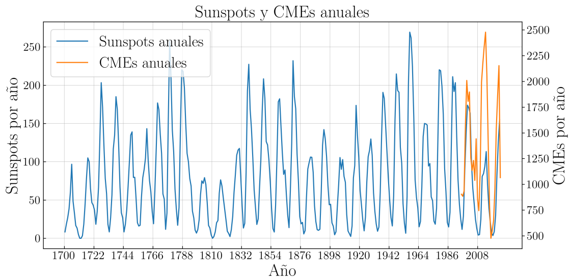
Figura 1.5: En el eje izquierdo se indica el perfil anual de la serie temporal de aparición de sunspots desde 1700 (curva azul), adaptado de la World Data Center for the Sunspot Index and Long-term Solar Observations (WDC-SILSO) 4 . En el eje derecho se muestra la cantidad de CMEs anuales desde 1996 (curva naranja), tomado de la base de datos SOHO-LASCO 5 , generada y mantenida en el Centro de Datos CDAW por la NASA y la Universidad Católica de América en cooperación con el Laboratorio de Investigación de la Marina. Figura de elaboración propia.
