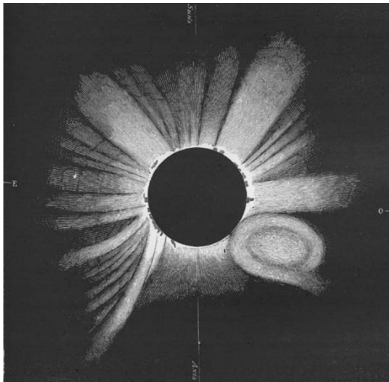
Figura 2.1: Dibujo del eclipse de 1860 registrado por Ernst Wilhelm Leberecht Tempel. Se piensa que esta es la primera observación de una eyección de masa coronal. Tomada de «Photographs and Drawings of the Corona» (1879).
