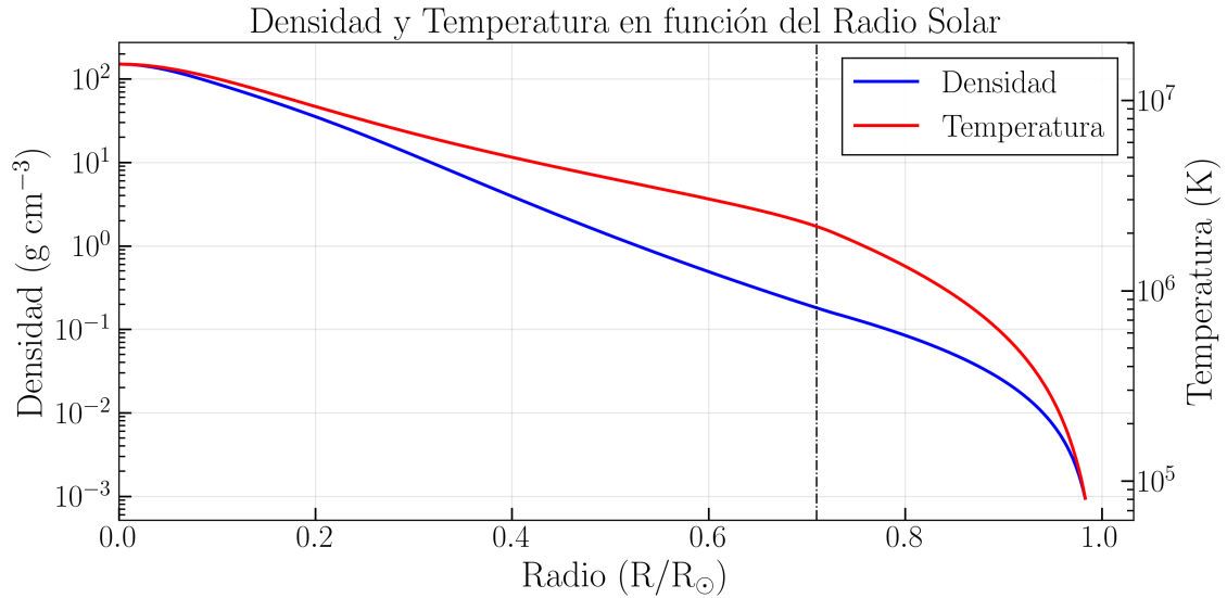
Figura 1.1: Distribución radial de densidad y temperatura en el modelo solar estándar interno. La densidad, en azul, muestra un decrecimiento de \sim 150 \text{ g cm}^{-3} en el centro a \sim 10^{-4} \text{ g cm}^{-3} en la superficie. La temperatura, en rojo, disminuye desde \sim 1,5 \times 10^7 K en el núcleo hasta \sim 5800 K en la fotosfera. La línea discontinua indica la ubicación de la tacoclina, en R = 0,71 R_{\odot} . Datos tomado de Software and Data for Solar Neutrino Research , véase nota 2 de pie de página 16. Figura de elaboración propia.
