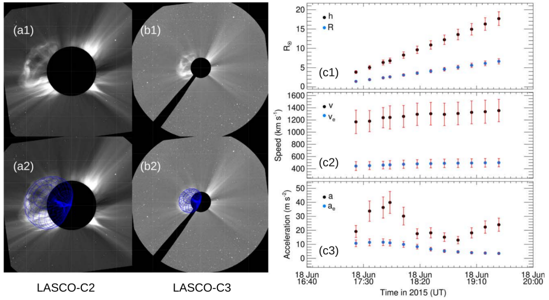
Figura 2.7: Imágenes de los coronógrafos LASCO-C2 (a1) y C3 (b1), del 18 de junio de 2015 en CR2165. Las imágenes a2 y b2 presentan los resultados de utilizar el modelo de cono elíptico (en azul), sobre la misma imagen a1 y b1. En el panel derecho se muestra la evolución de la altura ( h ), velocidad ( V ) y aceleración ( a ) de la CME en función del tiempo (puntos negros), además del ancho ( R ), la velocidad de expansión ( v_e ) y la aceleración de expansión ( a_e ) en función del tiempo (Mayank et al., 2023).
