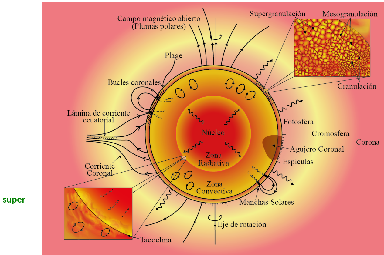
Figura 1.1: Esquema de la estructura interna y externa del Sol, mostrando sus principales capas físicas y fenómenos asociados. En el interior se distinguen el núcleo, la zona radiativa y la zona convectiva, separadas por la tacoclina ampliada en el panel inferior izquierdo. En la superficie solar aparecen la fotosfera, cromosfera y corona, junto con manifestaciones de la actividad magnética a través de manchas solares, espículas, granulación, bucles coronales, plages y plumas polares, estas últimas asociadas con líneas de campo magnético abiertas en agujeros coronales. Se muestran en el panel superior derecho los tipos de granulación: granulación, mesogranulación y supergranulación. También se ilustran estructuras coherentes extendidas como los corrientes coronales y la hoja de corriente ecuatorial. Las líneas de campo magnético se dibujan como líneas abiertas y cerradas suaves, mientras que la convección se muestra con flechas circulares en la zona convectiva; la emisión de fotones se indica con flechas onduladas en regiones como la zona radiativa y la fotosfera.
