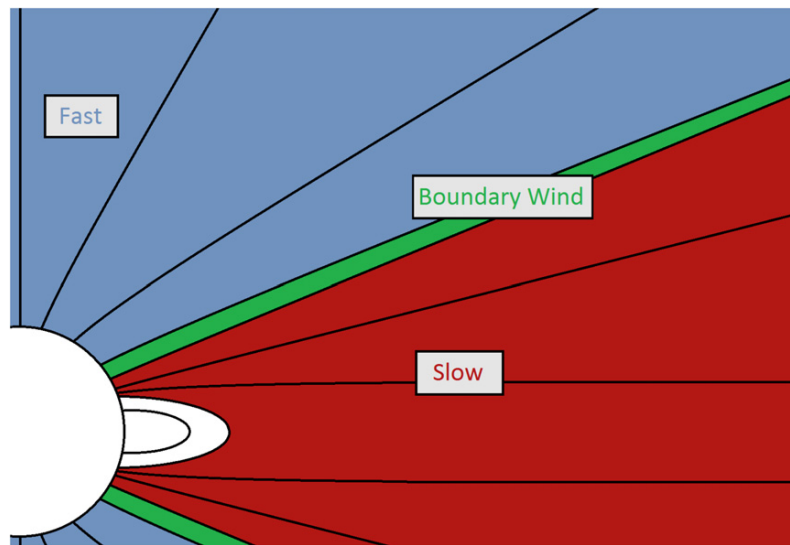
Figura 1.8: Diagrama de la distribución de los tipos de viento solar. En rojo está el viento lento, en azul el viento rápido y en verde el viento de interfaz. Tomado de Stakhiv et al. (2015).
