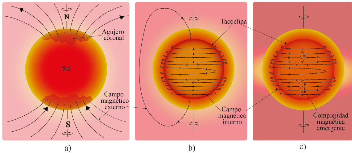
Figura 1.5: Comportamiento poloidal y toroidal del campo magnético del Sol. El panel a) muestra campos poloidales, un polo norte y un polo sur con líneas de campo magnético abiertas; el b) muestra su conversión interna en campos toroidales mediante el efecto \Omega , produciendo líneas de campo que envuelven el eje de rotación y sobre la tacoclina. El panel c) muestra el campo magnético emergente en forma de bucles a través de la superficie, regenerando el campo poloidal mediante el efecto \alpha .
