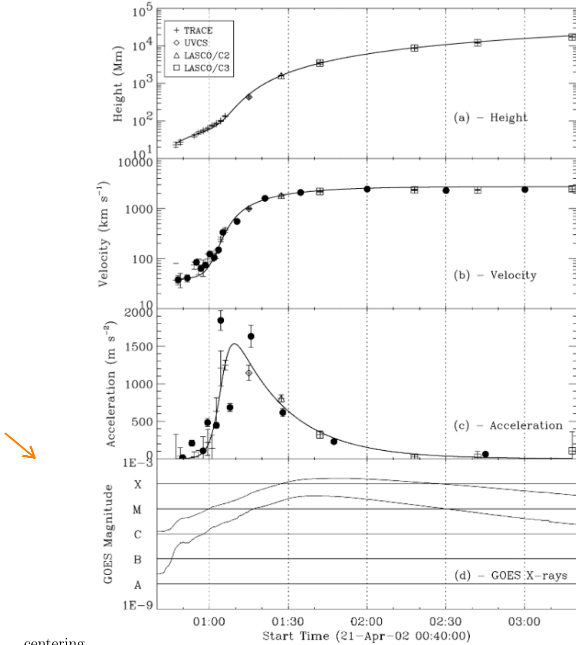
Figura 2.5: Perfil de altura, velocidad y aceleración de la CME del 21 de abril de 2002 a las 00:43 UT, en función del tiempo. Así mismo, el flujo de rayos X debido a su Flare asociada, en función del tiempo. Los círculos rellenos son valores derivados de la gráfica de altura vs tiempo, los demás símbolos señalan las observaciones del TRACE, UVCS y del LASC0. La línea continua indica la curva con el mejor ajuste para los datos. (Gallagher et al., 2003).
