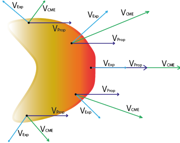
Figura 2: Representación de los vectores velocidad de propagación ( V_{\text{Prop}} ) y de expansión ( V_{\text{Exp}} ) en puntos cualquiera de la CME. El vector V_{\text{Exp}} presenta direcciones hacia fuera de la CME en diferentes puntos, mientras que el vector V_{\text{Prop}} tiene una dirección hacia la derecha en todo punto de la CME. Además, el vector resultante de la superposición del vector propagación y expansión, se muestra como V_{\text{CME}} y cambia de dirección según el punto dentro de la CME.
