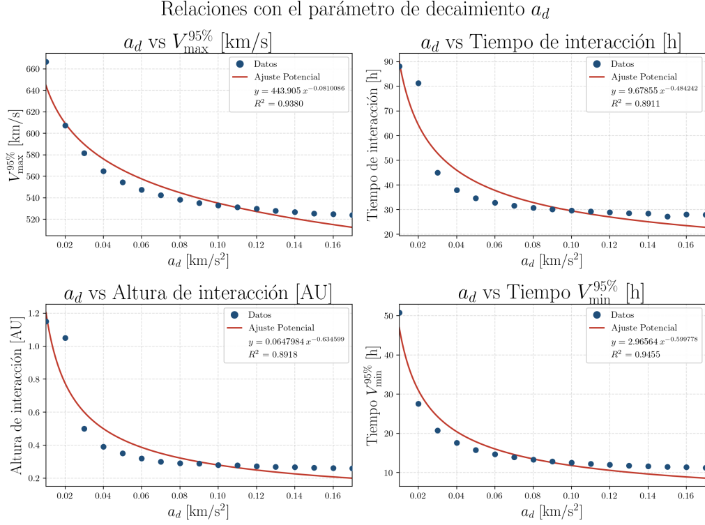
Figura 4.5: Gráficas de a_d vs parámetros de interacción, junto a las curvas de ajuste (línea roja) correspondientes y sus ecuaciones características. Los puntos en azul son los datos de la CME sucesora bajo los cuales ocurre la interacción. Además, se muestra su coeficiente de correlación.
