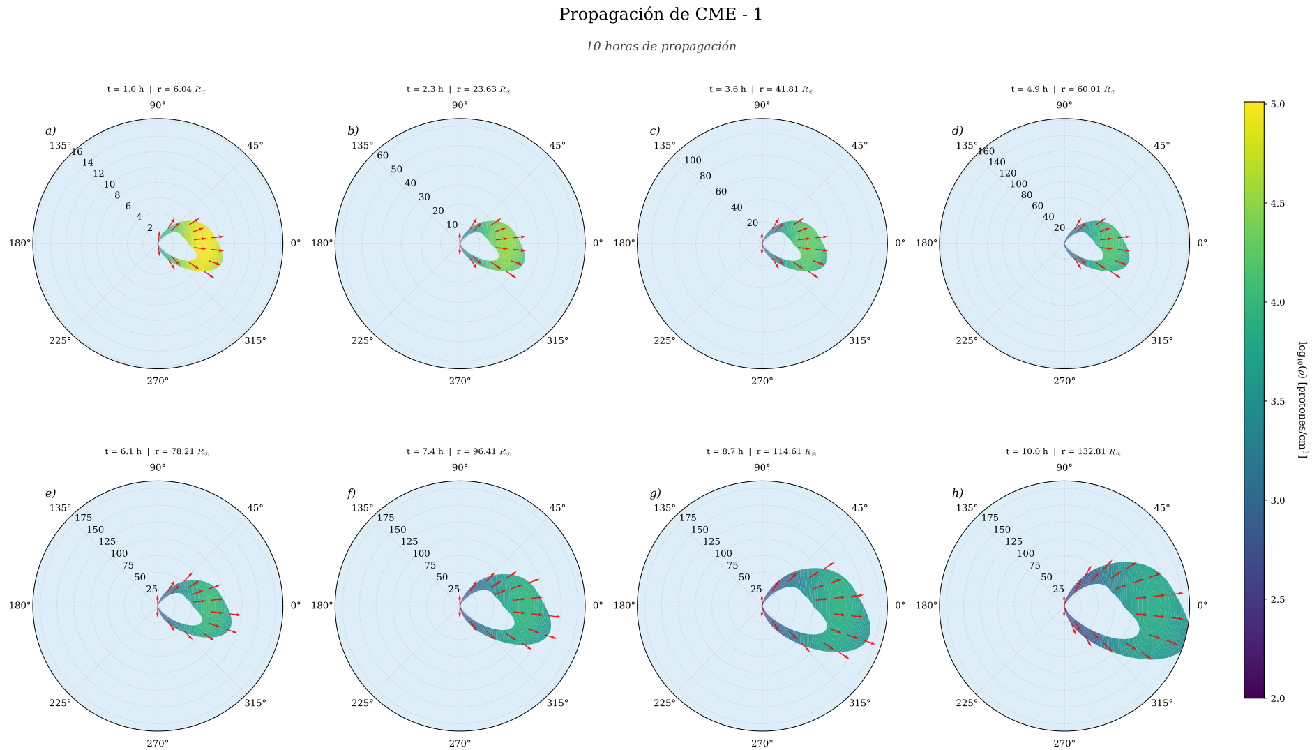
Figura 4.4: Evolución en 2D de la CME-1 durante 10 horas. La densidad se describe en escala de colores y la velocidad a través de un campo vectorial en rojo. En la parte superior de cada panel se indica el tiempo transcurrido y la posición del centro de la CME.
