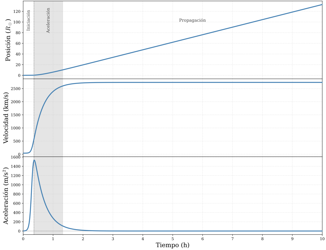
Figura 4.3: Perfiles de posición, velocidad y aceleración para la simulación de la CME inicial. Las diferentes etapas en la evolución de la CME se identifican con regiones delimitadas; la región de iniciación se indica en blanco hasta la línea discontinua, la etapa de aceleración se muestra en gris desde la línea discontinua hasta la punteada, la región de propagación en blanco va desde la línea punteada hasta el final de la gráfica. La línea discontinua indica el momento en el que la aceleración es máxima, mientras que la línea punteada señala el momento en el que la velocidad alcanza el 95 % de su velocidad máxima. Cabe señalar que el punto que se toma para determinar la cinemática de la CME es en su centro.
