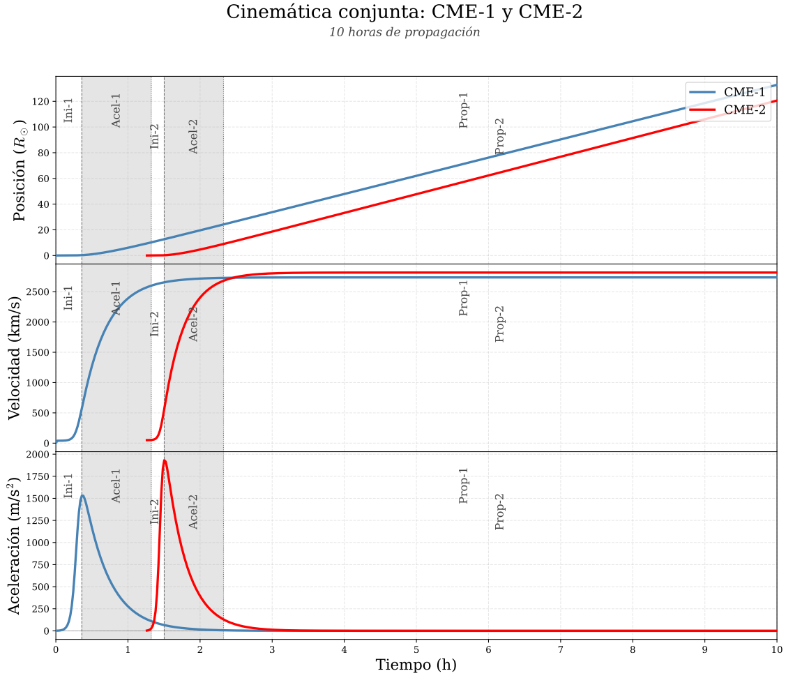
Figura 4.7: Perfiles cinemáticos de las dos CMEs sin considerar interacción. En azul se muestra la cinemática de la CME-1 y en rojo la de la CME-2, además se señalan las regiones de iniciación (blanco), aceleración (gris) y propagación (blanco) de las CMEs, etiquetadas con Ini, Acel y Prop. También, las etapas de iniciación y aceleración están separadas por una línea discontinua, mientras que las etapas de aceleración y propagación lo están con una línea punteada.
