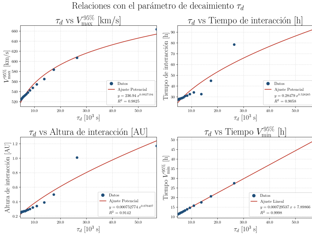
Figura 4.11: Gráficas de \tau_d vs parámetros de interacción, junto a las curvas de ajuste (línea roja) correspondientes y sus ecuaciones características. Los puntos en azul son los datos de la CME sucesora bajo los cuales ocurre la interacción. Además, se muestra su coeficiente de correlación.
