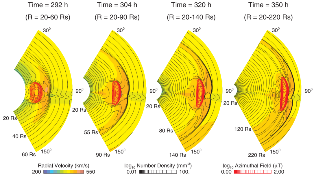
Figura 2.2: Propagación de una CME en la heliosfera, en donde la escala de colores muestra el mapa de velocidades, la densidad del plasma se muestra en relación a la densidad de líneas negras y el campo magnético en relación a la densidad de líneas rojas. Se muestra la evolución de la CME en 4 tiempos: 292, 304, 320 y 350 horas después de empezar a correr la simulación
