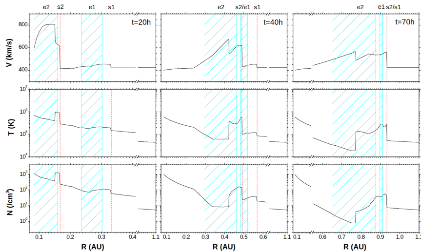
Figura 3.3: Resultados de la simulación a 1D, con intervalos de tiempo diferentes, donde e1 y e2 son la primera y segunda CME, respectivamente; s1 y s2 son las ondas de choque de las CMEs 1 y 2, respectivamente.
