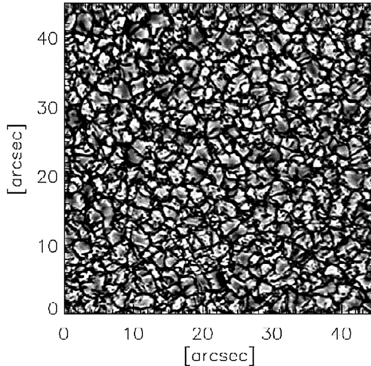
Figura 1.4: Imagen de intensidad del continuo a 5250.4 \text{ \AA} obtenida con el instrumento IMaX a bordo del telescopio Sunrise I (junio de 2009). Se observa el patrón de granulación solar, donde las estructuras brillantes corresponden a celdas convectivas de plasma caliente ascendente (gránulos), delimitadas por carriles intergranulares oscuros de material descendente y más frío. El campo de visión abarca aproximadamente 35 \times 35 \text{ Mm} con una resolución espacial de \sim 100 \text{ km} por píxel. Adaptado de Solanki et al. (2010).
