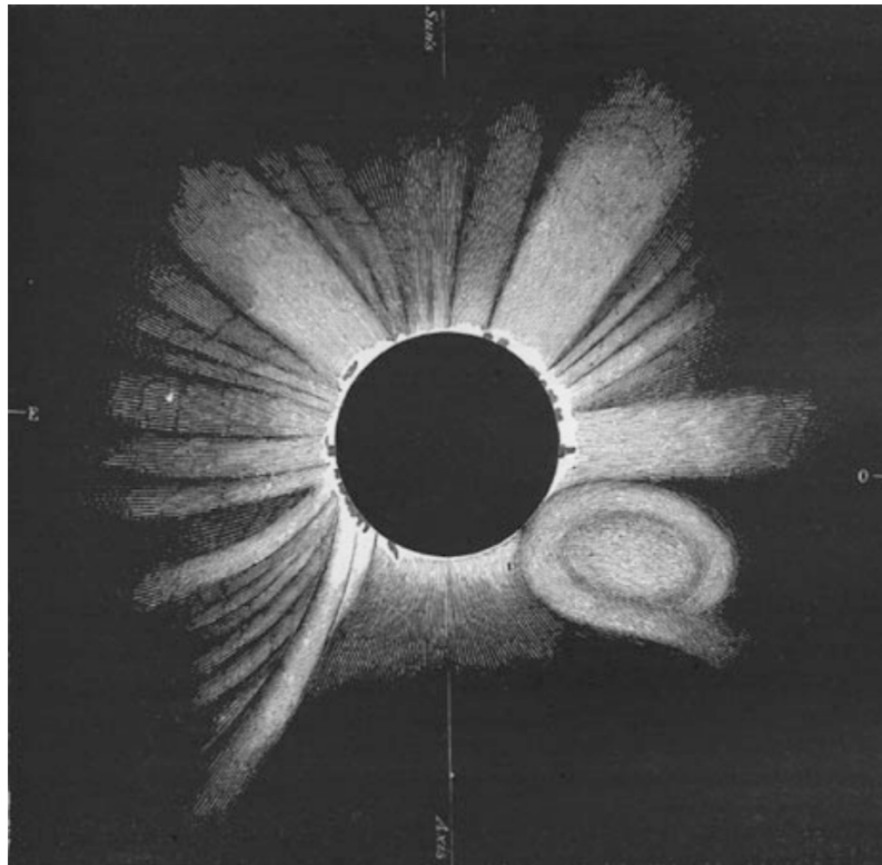
Figura 1.1: Dibujo del eclipse de 1860 registrado por Tempel, «Photographs and Drawings of the Corona», 1879 . Se piensa que esta es la primera observación de una eyección de masa coronal.
