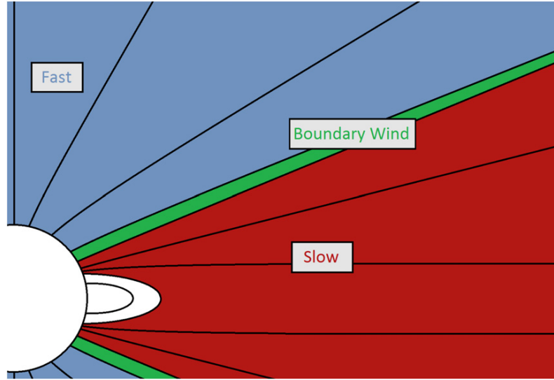
Figura 1.2: Diagrama del viento solar, en rojo el viento lento, en azul el viento rápido, en verde el viento de interfaz, extraído de Stakhiv et al., 2015.
