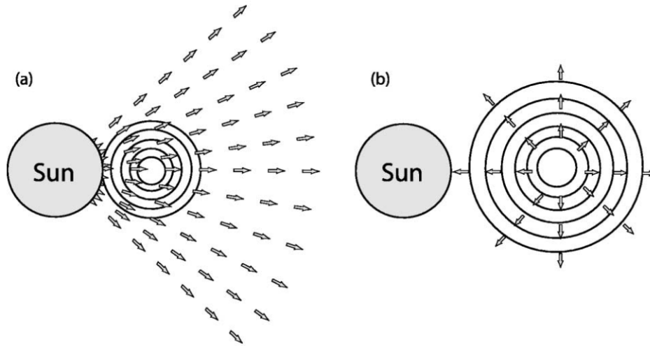
Figura 2.1: Efectos cinematicos en la evolución de la CME. En a) se muestra la evolución convectiva o expansión esférica; y en b) se muestra la expansión de la CME causada por un gradiente de presión entre ella y el viento solar ambiental, Riley y Crooker, 2004.
