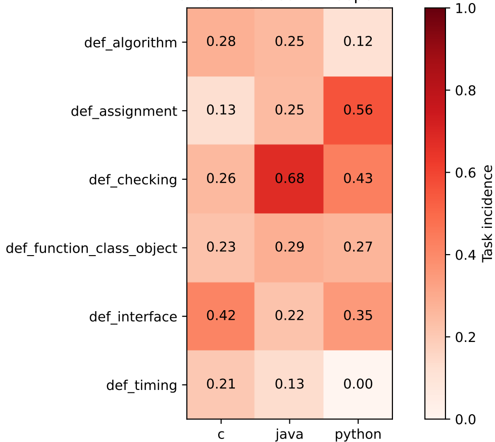
ODC incidence — DeepSeek
