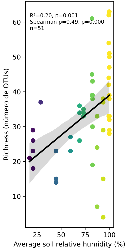
Richness (número de OTUs)
