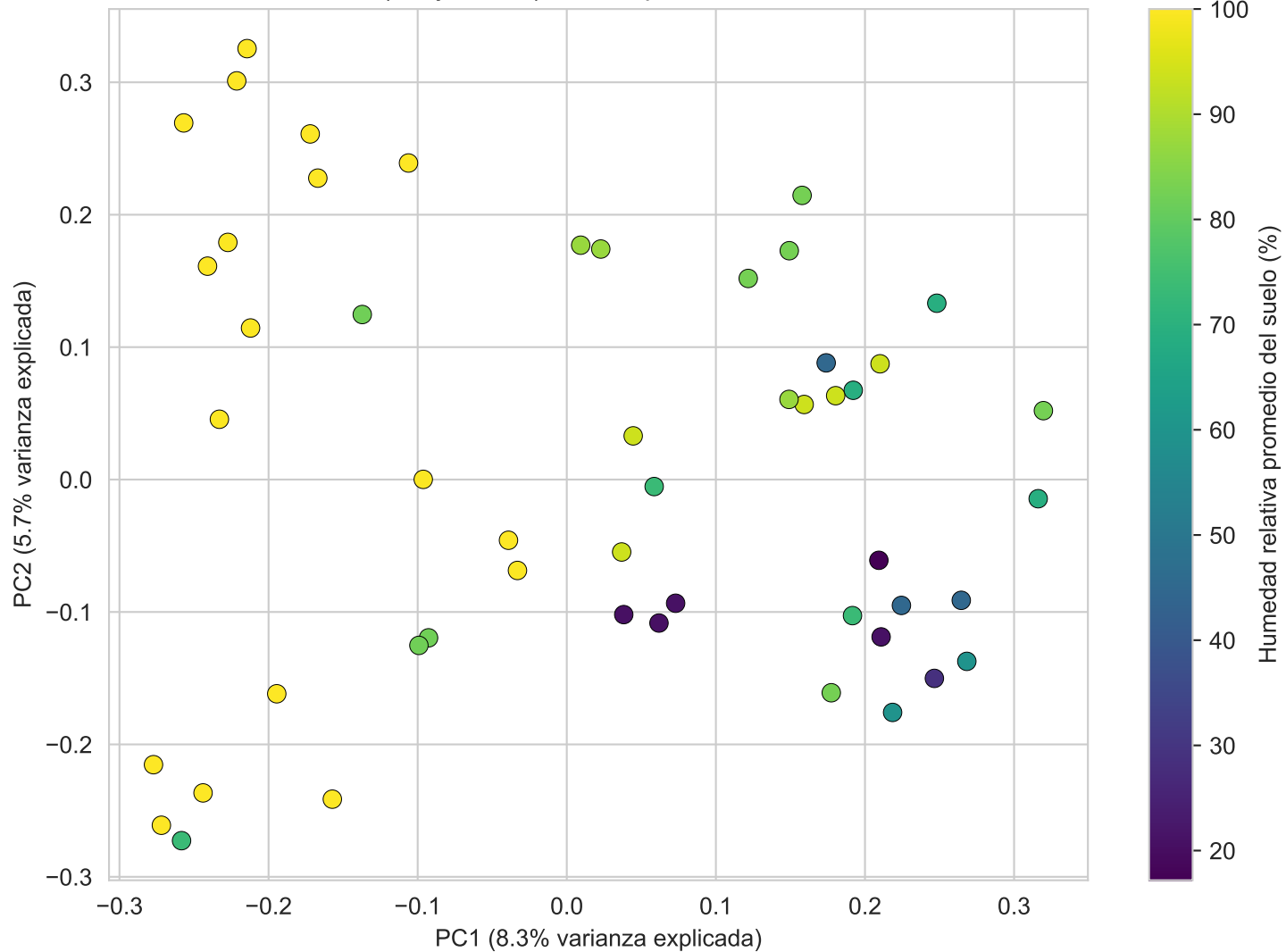
PCoA (Bray-Curtis) de composicion microbiana
