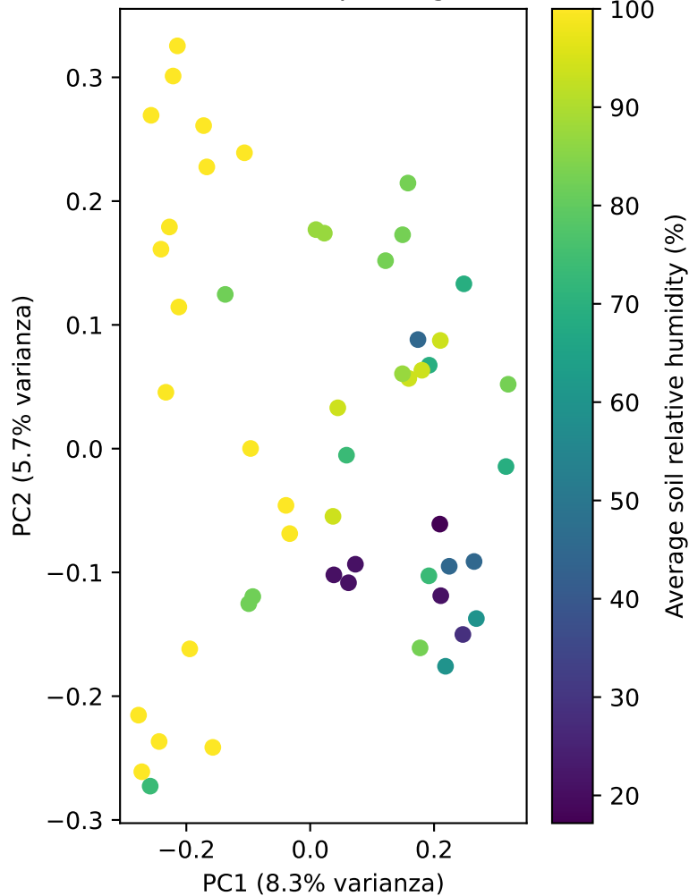
PCoA coloreado por AvgSoilRH
