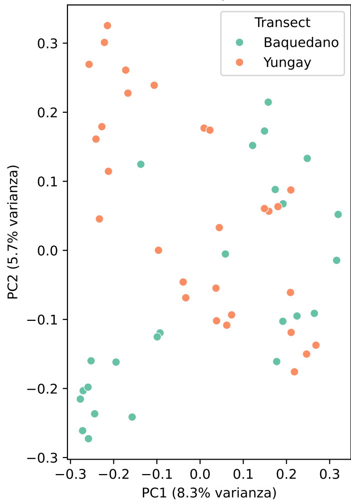
PCoA coloreado por transecto
