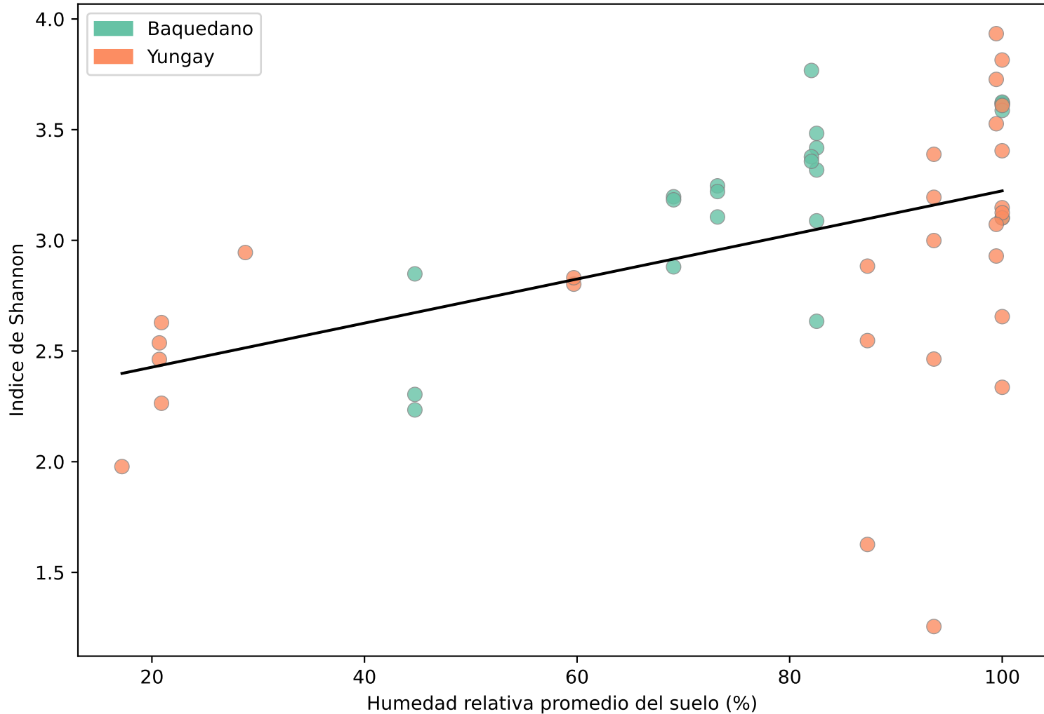
Diversidad alfa vs. humedad del suelo Spearman rho = 0.47, p = 0.0005, R2 = 0.21
