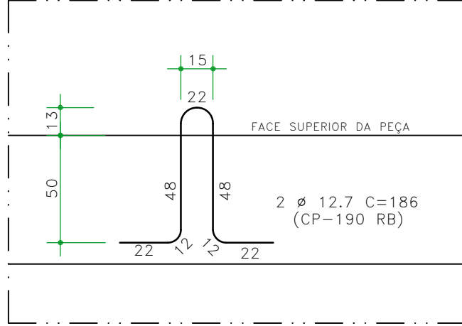
DETALHE ALÇA
