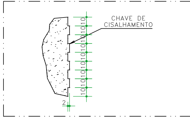
DETALHE 1
