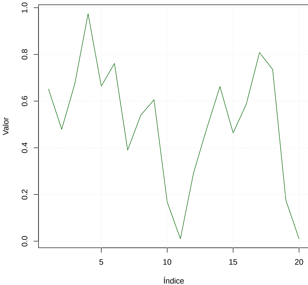
Gráfico Aleatorio 17
