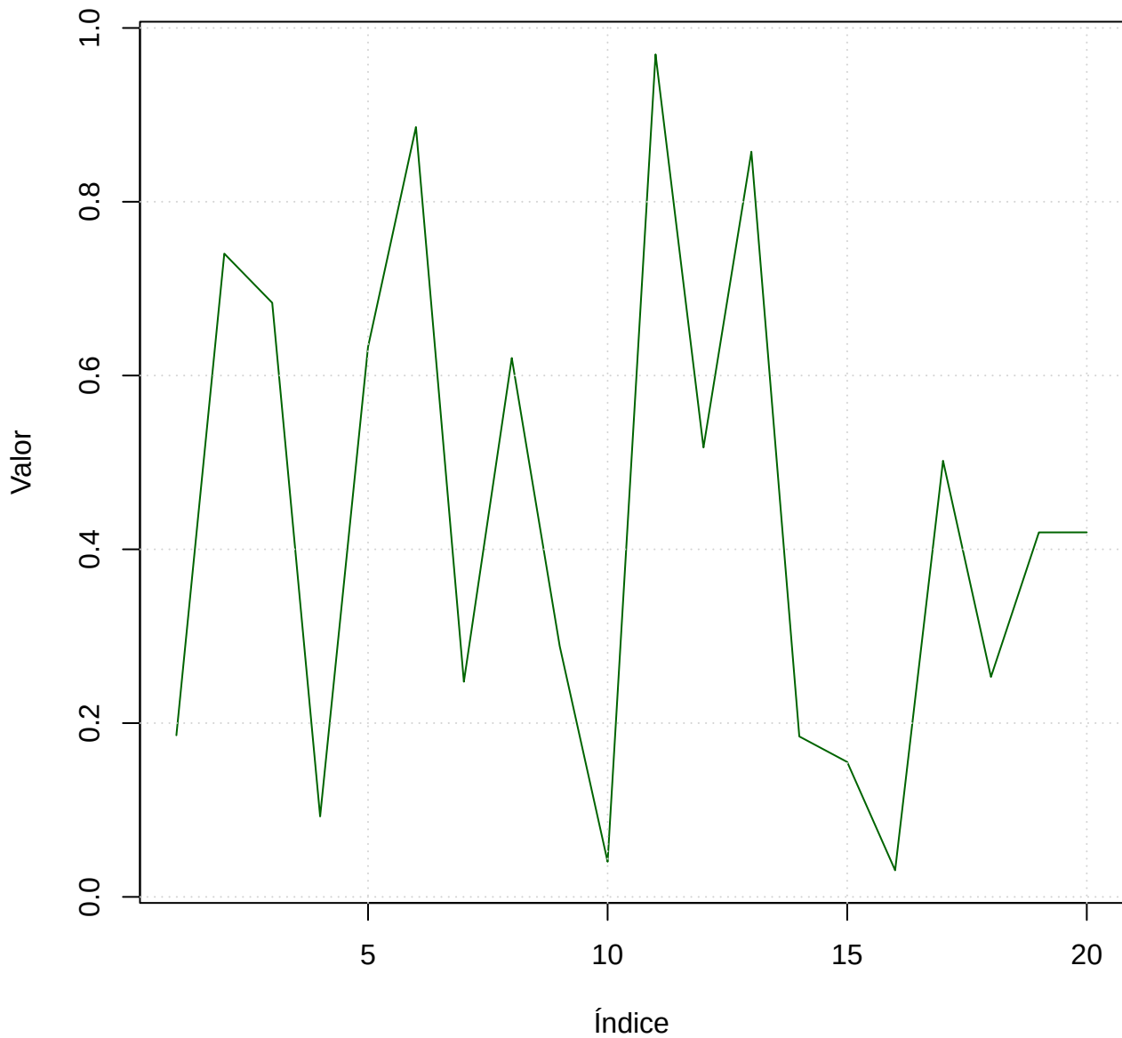
Gráfico Aleatorio 34
