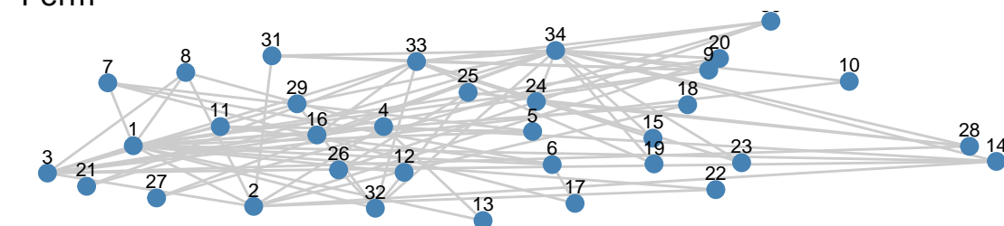
* Rand
