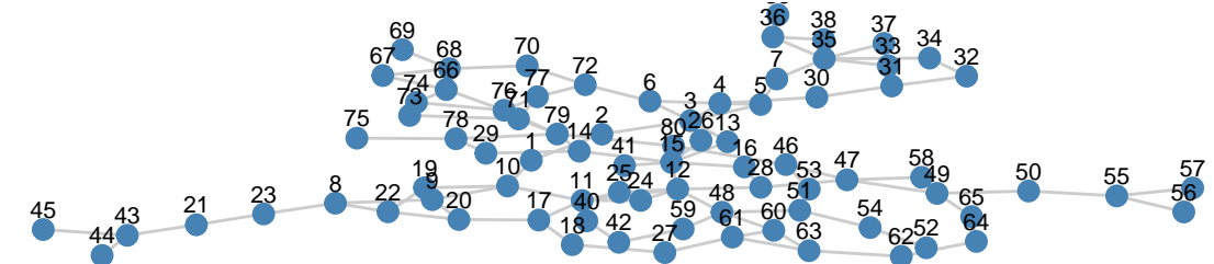
* Shift
