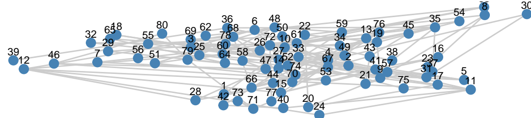
* Rand
