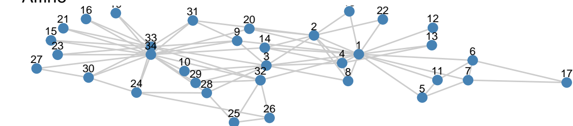
* Shift
