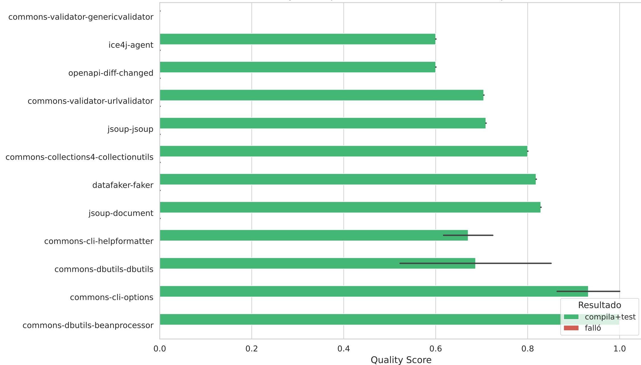
Quality score por dataset (con estado de compilación)
