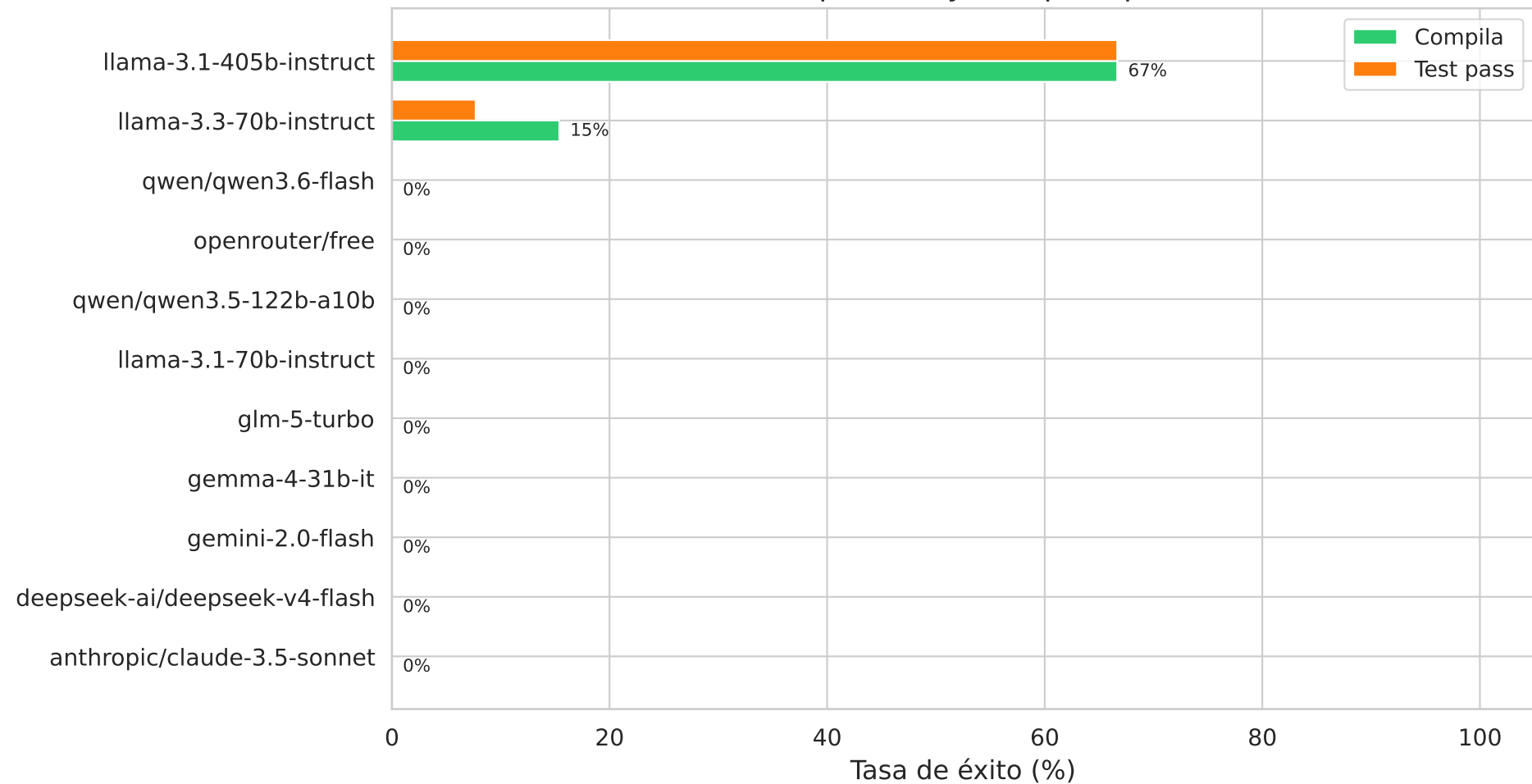
Tasa de compilación y test pass por modelo
