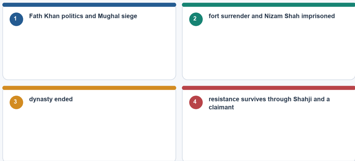
Daulatabad, 1633
