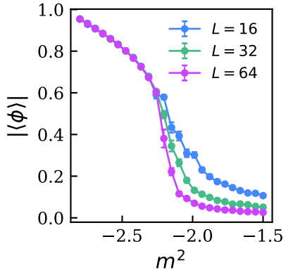
Order Parameter
