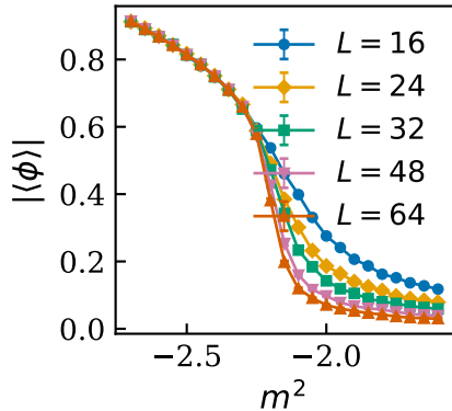
Order Parameter
