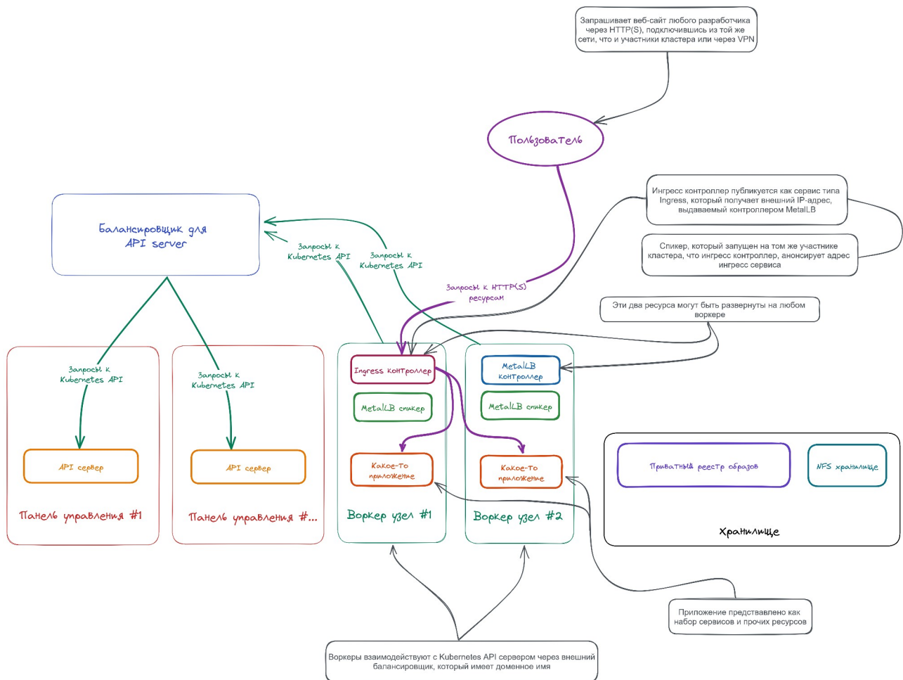
Рисунок 7 — Схема архитектуры кластера
