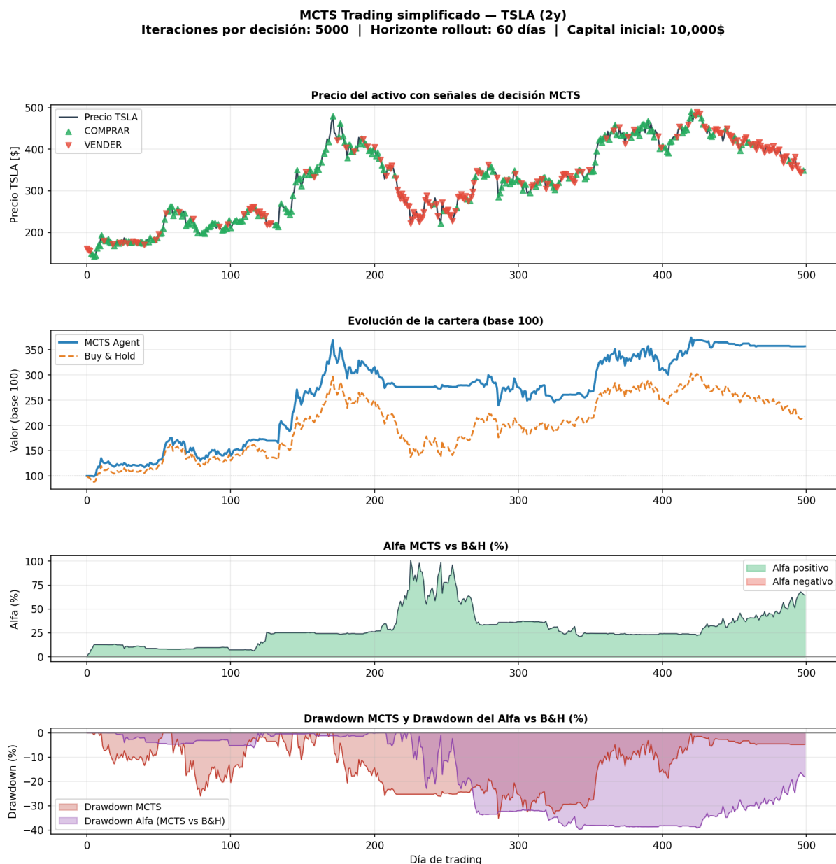
Figura 2: Panel de resultados. De arriba abajo: (1) precio de TSLA con señales COMPRAR/VENDER; (2) evolución de la cartera (base 100) MCTS vs. B&H; (3) alfa relativa MCTS vs. B&H; (4) drawdown de la cartera MCTS (rojo) y drawdown del alfa (morado).
