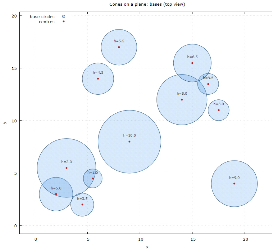
Рисунок 1. Вид сверху: основания конусов на плоскости
