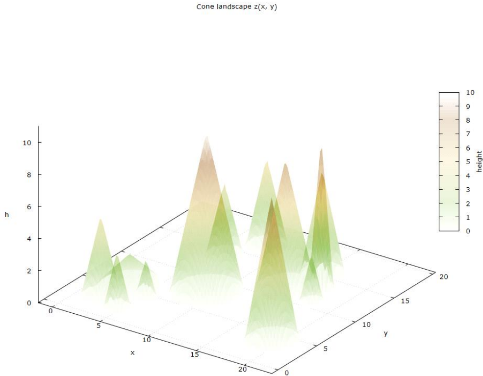
Рисунок 2. Ландшафт z(x, y) : поверхность конусов над плоскостью
