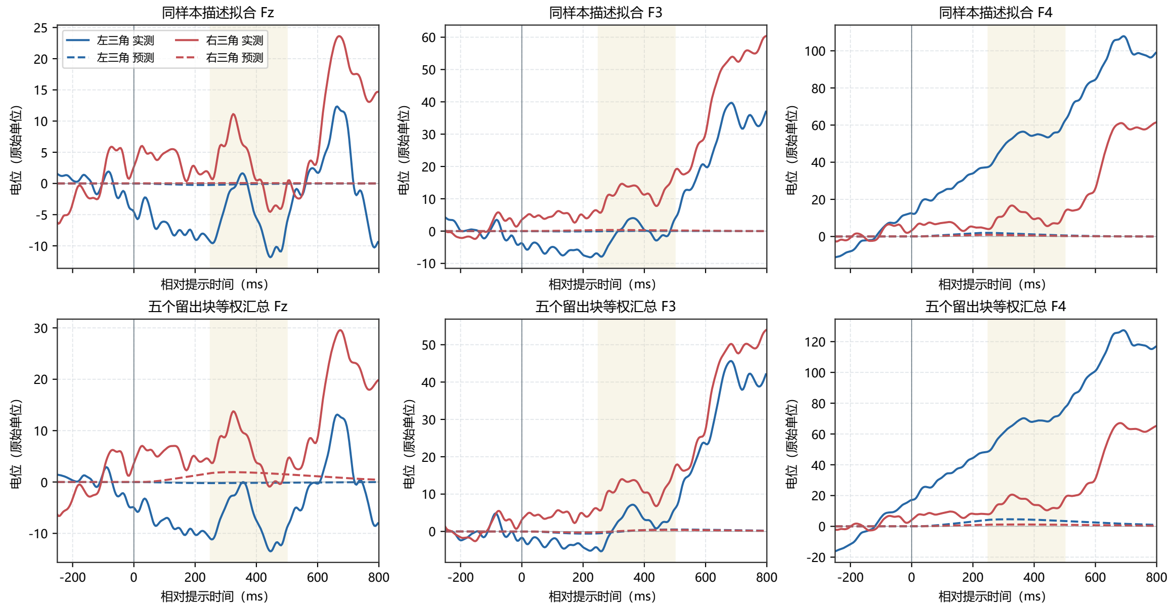
图3 B1组左右三角ERP拟合与留出预测
