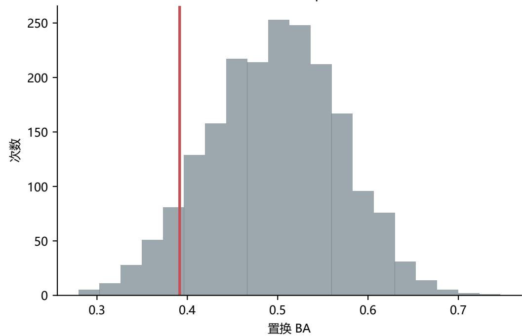
块内置换: maxT p=1.000
