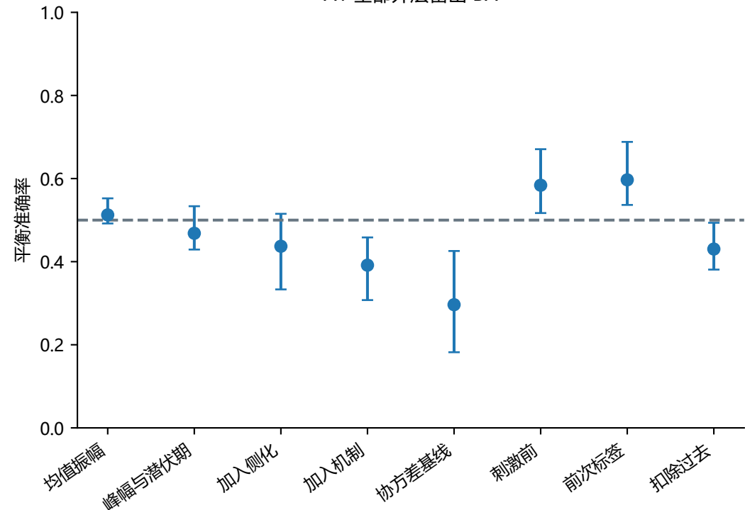
块内置换: maxT p=1.000
