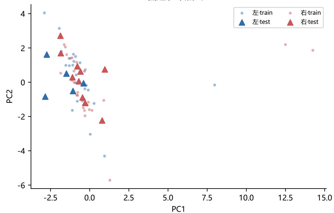
A1 固定第5块留出 PCA
