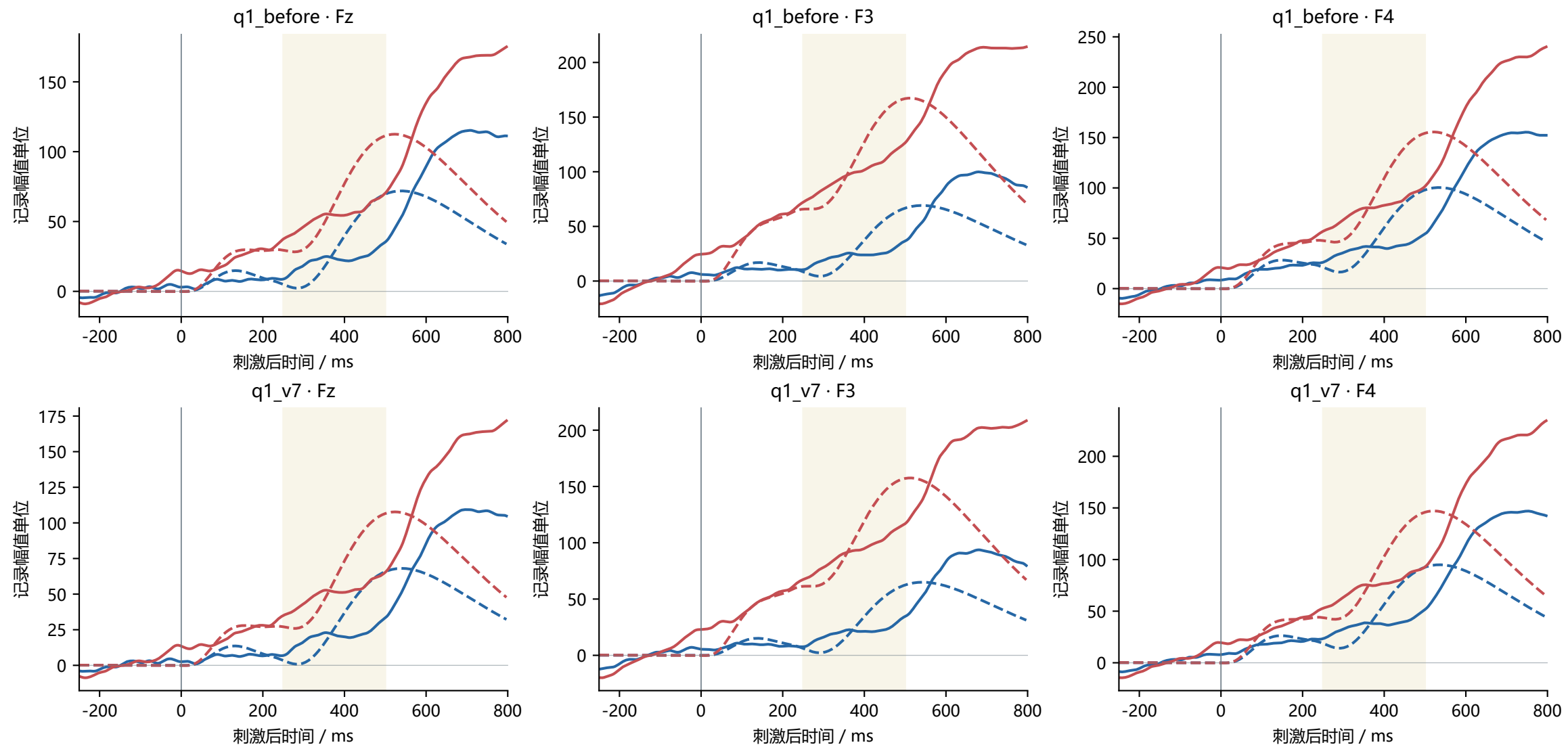
A2 Q1 衔接：实线为条件均值，虚线为同样本描述拟合（不计入预测证据）
