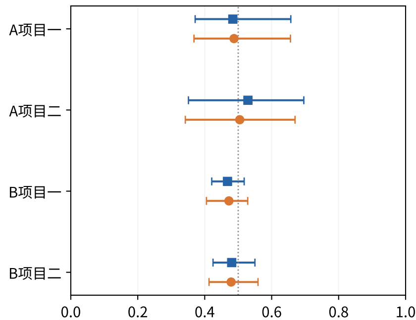
ROC AUC
