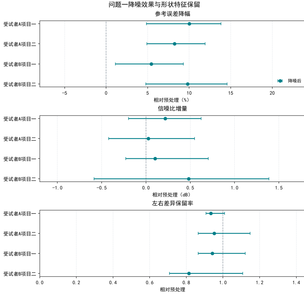
图 4.2 去噪性能与条件差异保留
