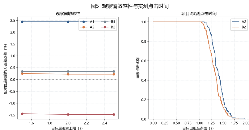
图 4.17 观察窗敏感性与点击时间分布
