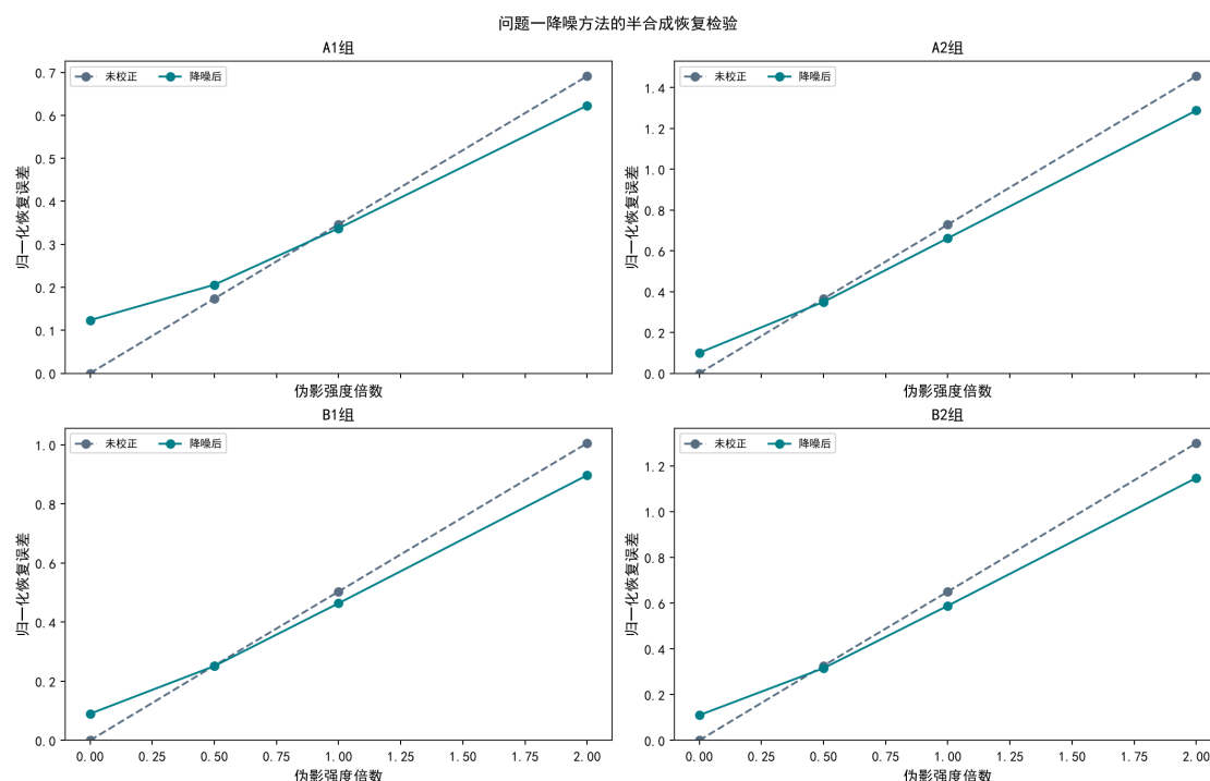
图 4.5 半合成伪影恢复结果
