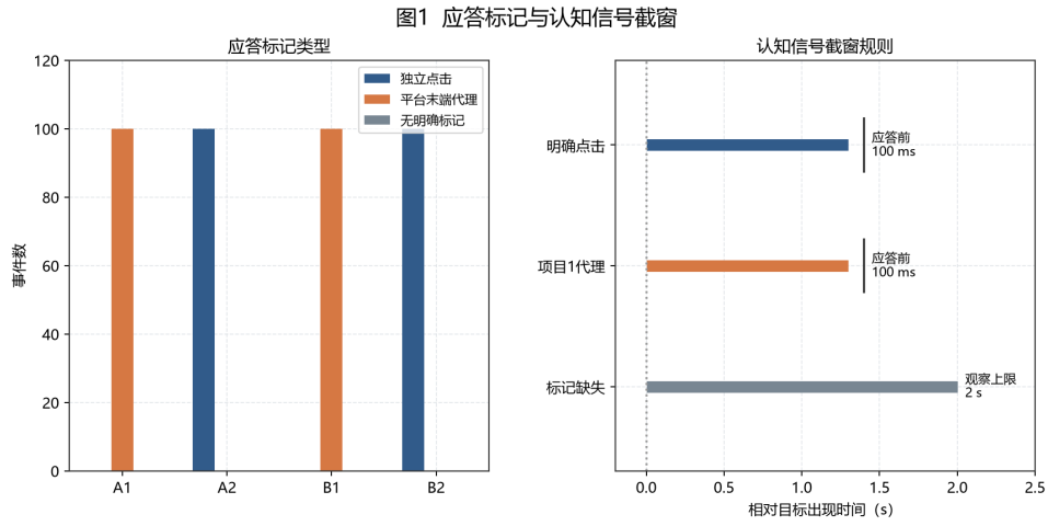
图 4.13 应答标记与认知信号截窗
