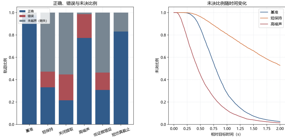
图 4.16 认知状态驱动的决策仿真图
