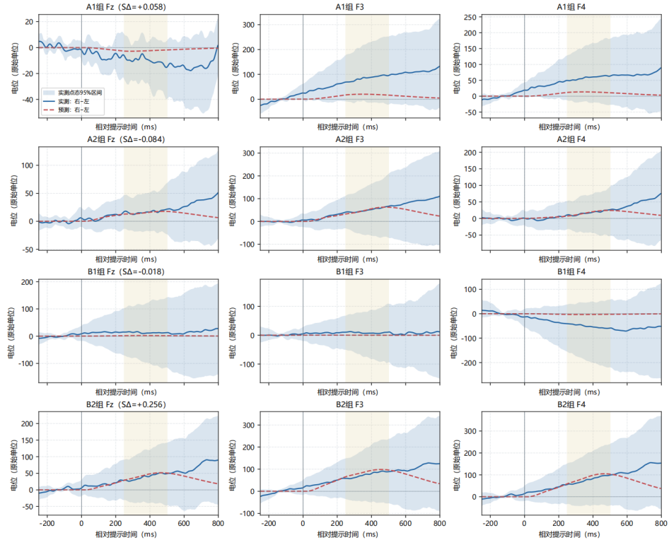
图 4.9 四组记录的 ERP 差异波预测图
