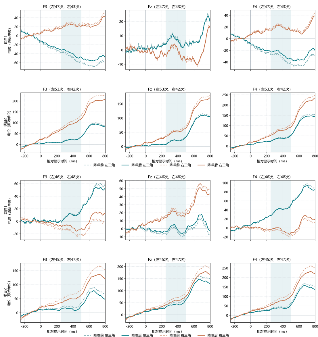
图 4.4 四组记录的三通道 ERP 图
