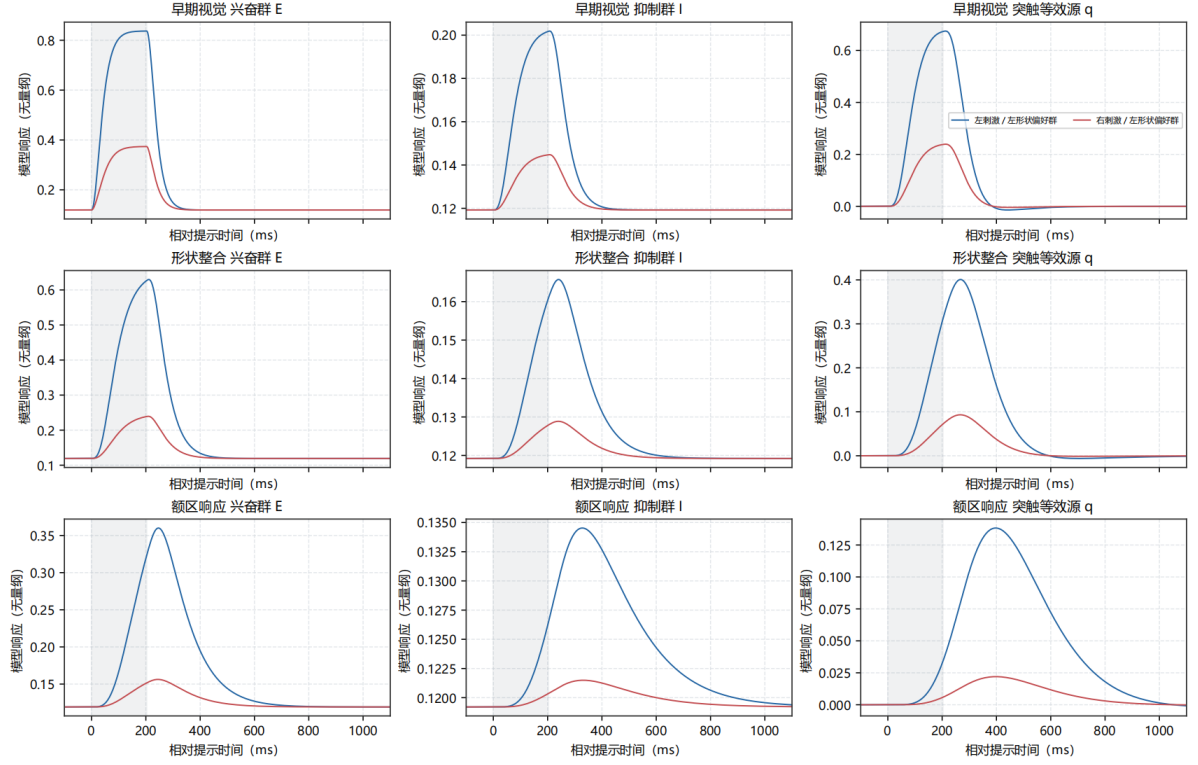
图 4.7 A1 三级神经群与等效源响应图
