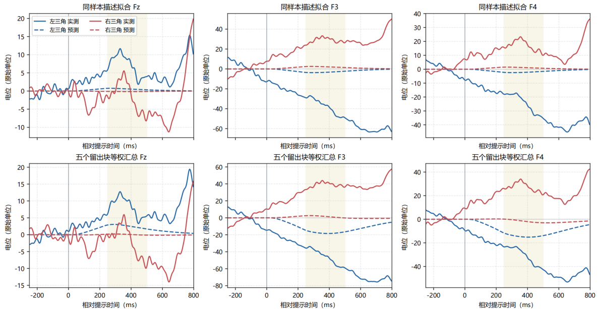
图 4.8 A1 ERP 拟合与留出预测图
