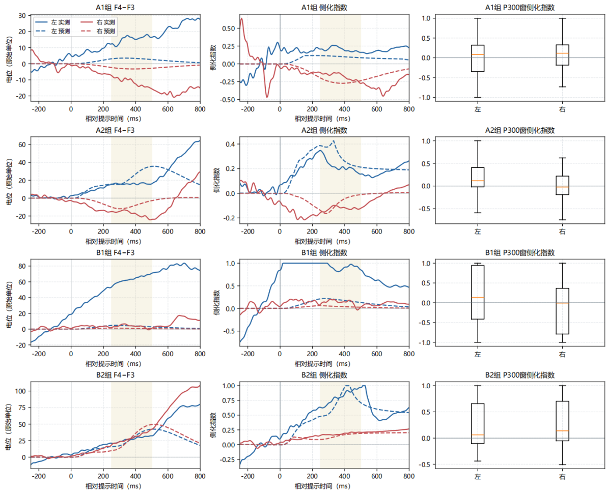
图 4.10 额区电位差与侧化指数图
