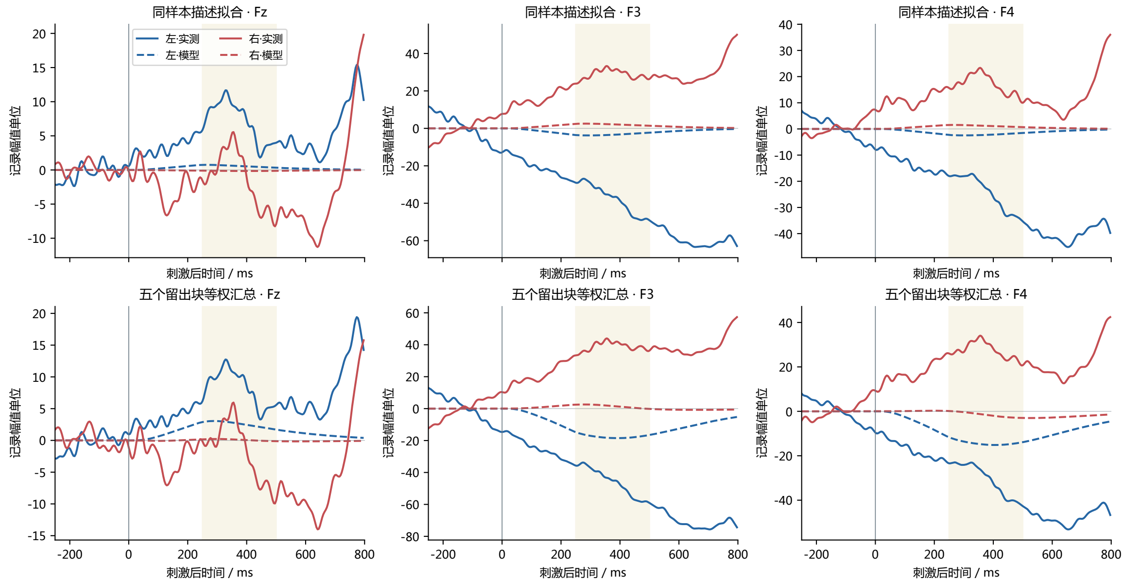
图3 A1 左右 ERP 的描述拟合与独立时间块预测
