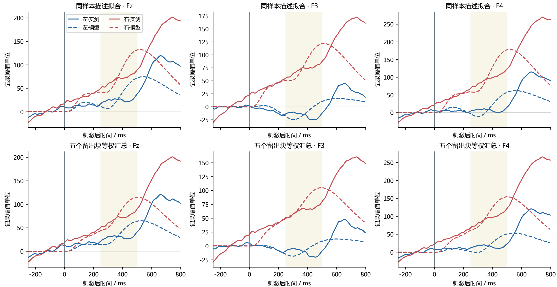
图3 B2 左右 ERP 的描述拟合与独立时间块预测
