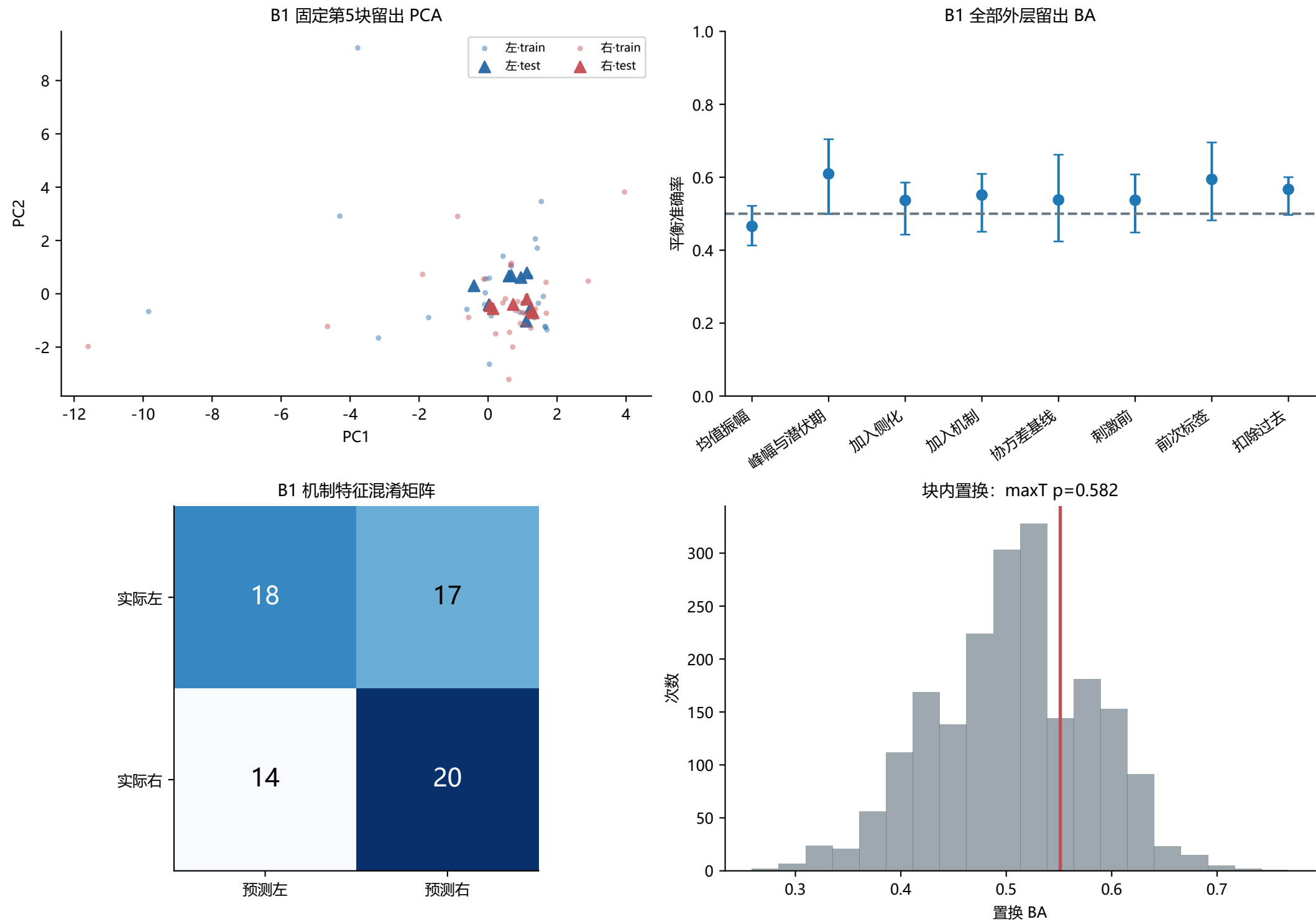
图7 B1 特征可视化与未知方向判别 (二维散点不作为显著性证据)
