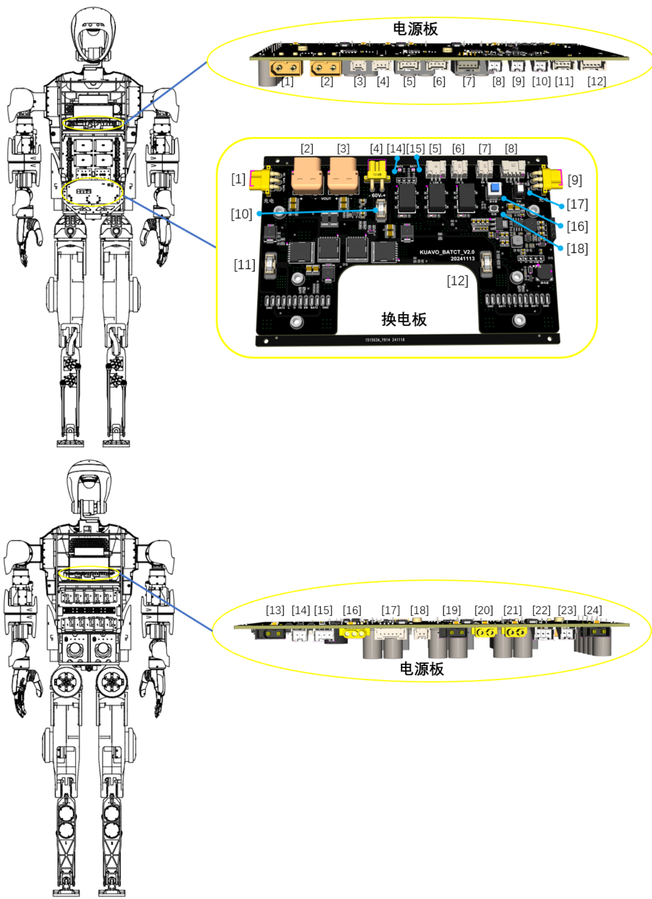
KUAVO_4pro_长手版电气接口
