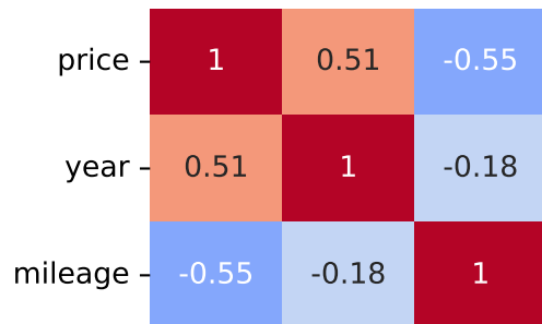
Pearson Correlation - Model: grande punto | Fuel: 2
