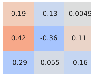
Pearson Correlation - Model: grande punto | Fuel: 5
