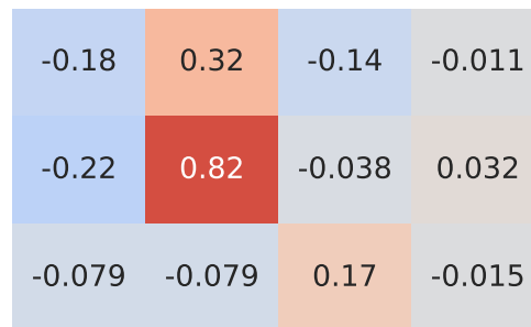
Pearson Correlation - Model: grande punto | Fuel: 4
