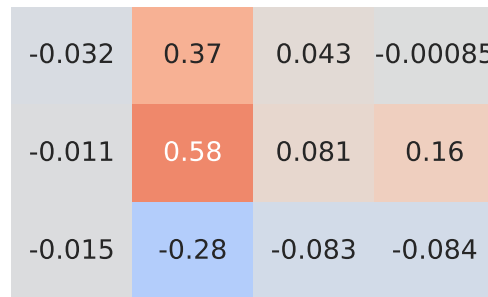
Pearson Correlation - Model: grande punto | Fuel: 1
