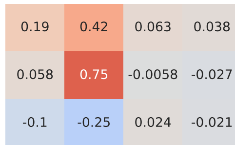
Pearson Correlation - Model: grande punto | Fuel: 2
