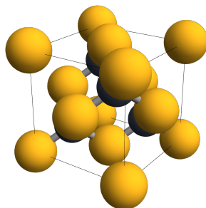
\text{S}^{2-} (黄) 与 \text{Zn}^{2+} (灰), \text{Zn}^{2+} 位于 \text{S}^{2-} 四面体空隙
