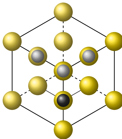
\text{S}^{2-} (黄) 与 \text{Zn}^{2+} (灰黑), \text{Zn}^{2+} 位于 \text{S}^{2-} 四面体空隙
