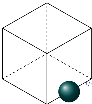
棱上：被 4 个晶胞共用（1/4）
