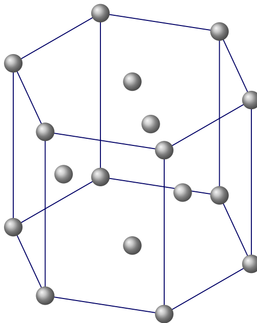
六方最密堆积晶胞（ABAB...，代表金属：Mg、Zn、Ti）
