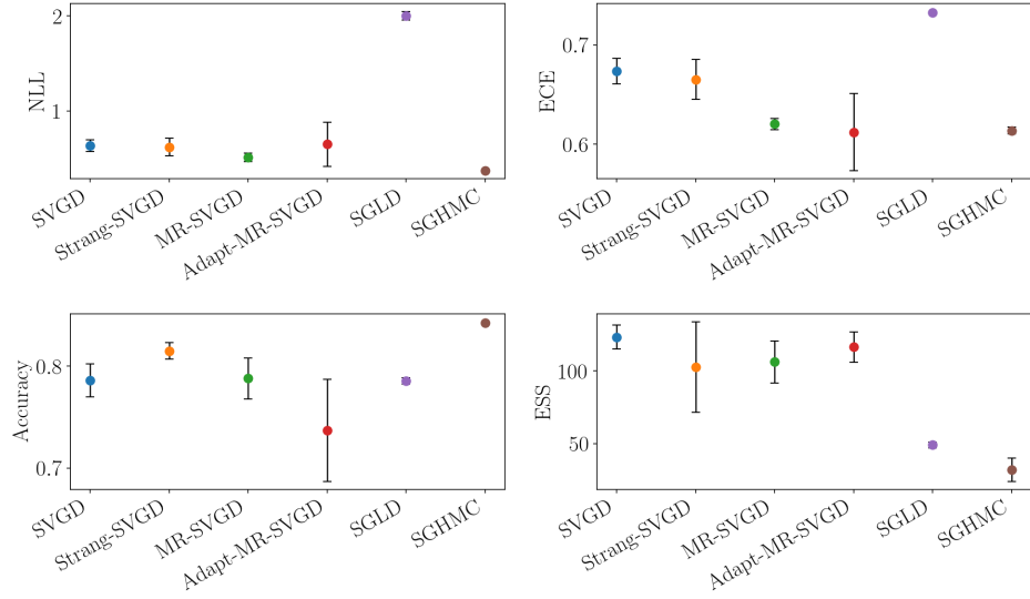
(d) a5a
