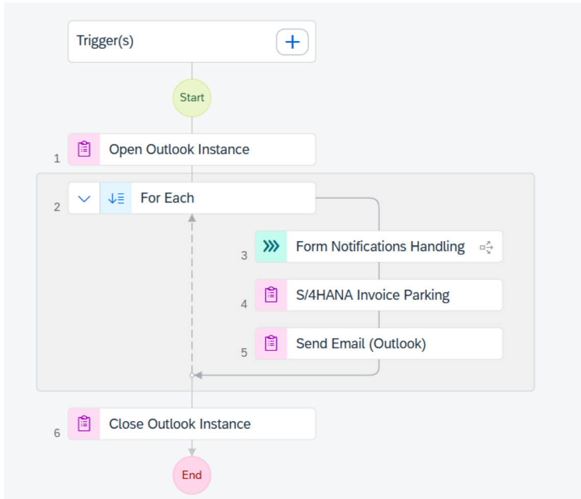
4.7. ábra. A folyamatlezáró és könyvelő automatizáció logikai felépítése
