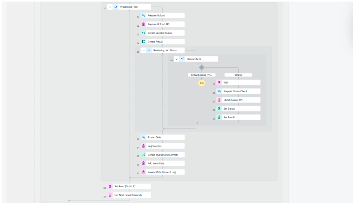
4.3. ábra. Az aszinkron feldolgozás státuszát figyelő ciklus (Polling Loop) implementációja
