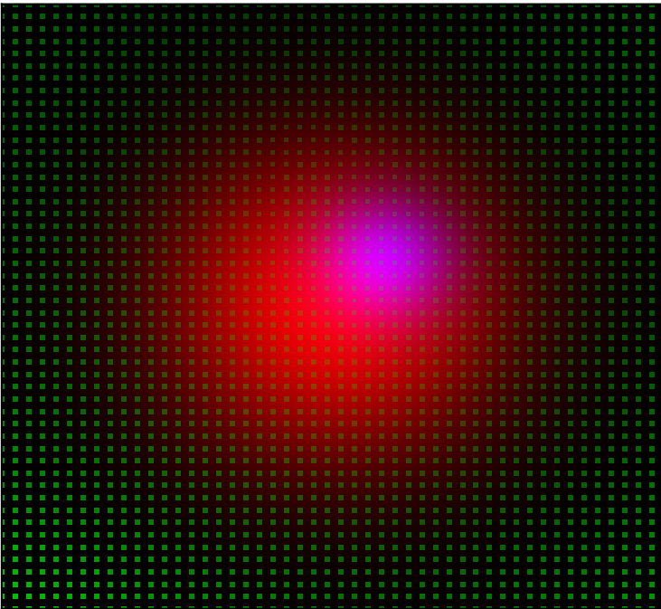
TSM (MAE: 37.122)
