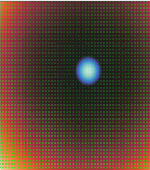
TSM (MAE: 37.122)
