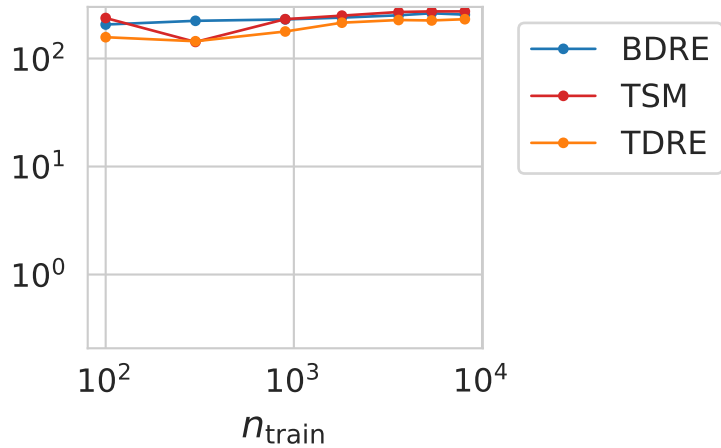
KL(p_0 \| p_1) = 32.4
