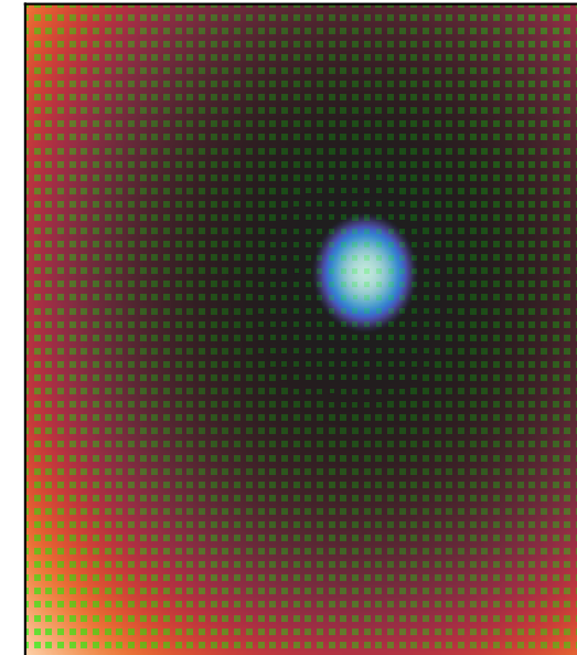
VFM (MAE: 30.008)
