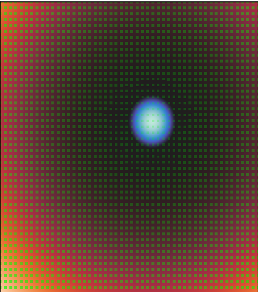
TDRE_5 (MAE: 33.976)
