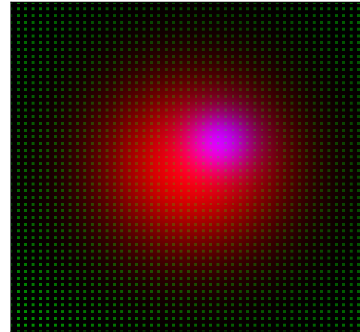
VFM (MAE: 30.008)
