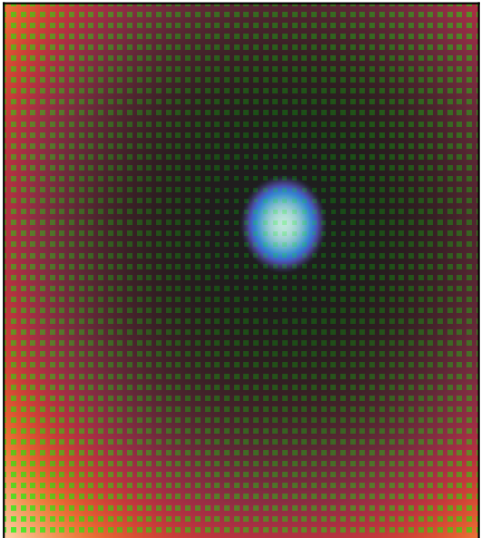
BDRE (MAE: 36.182)
