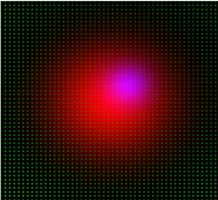
TDRE_5 (MAE: 33.976)
