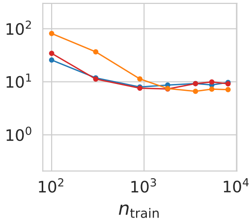
KL(p_0 \| p_1) = 5.4
