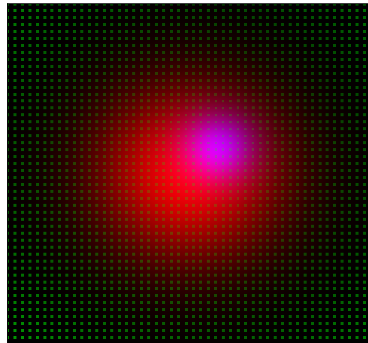
VFM (MAE: 30.008)
