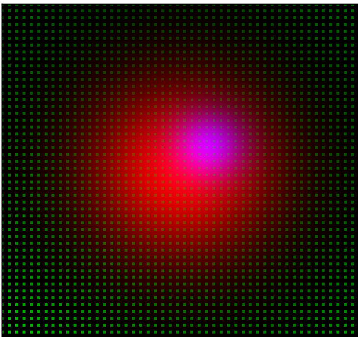
TSM (MAE: 37.122)
