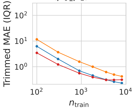
KL(p_0 \| p_1) = 0.6
