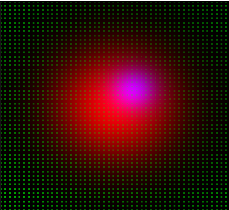
BDRE (MAE: 36.182)
