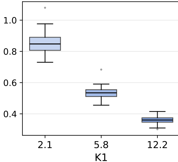
hill_tail
