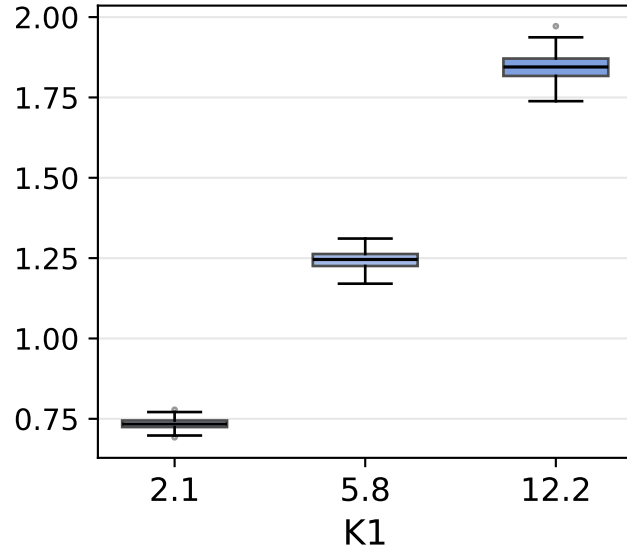
lip_q90
